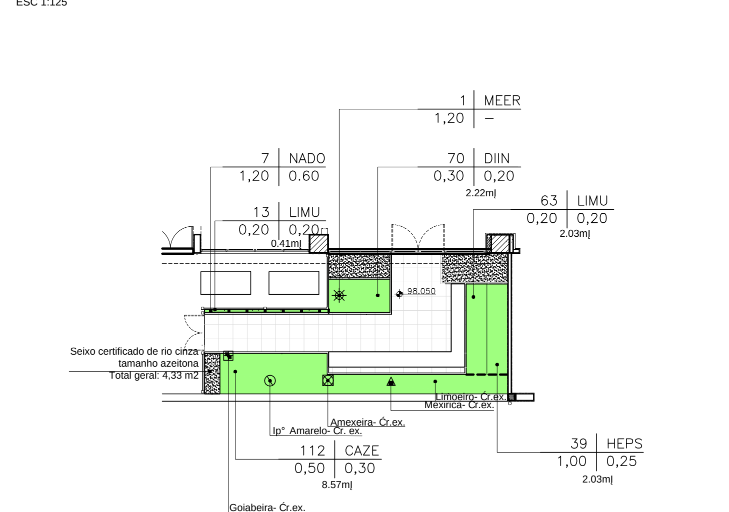
PLANTA - Jd. lateral A ESC 1:125
