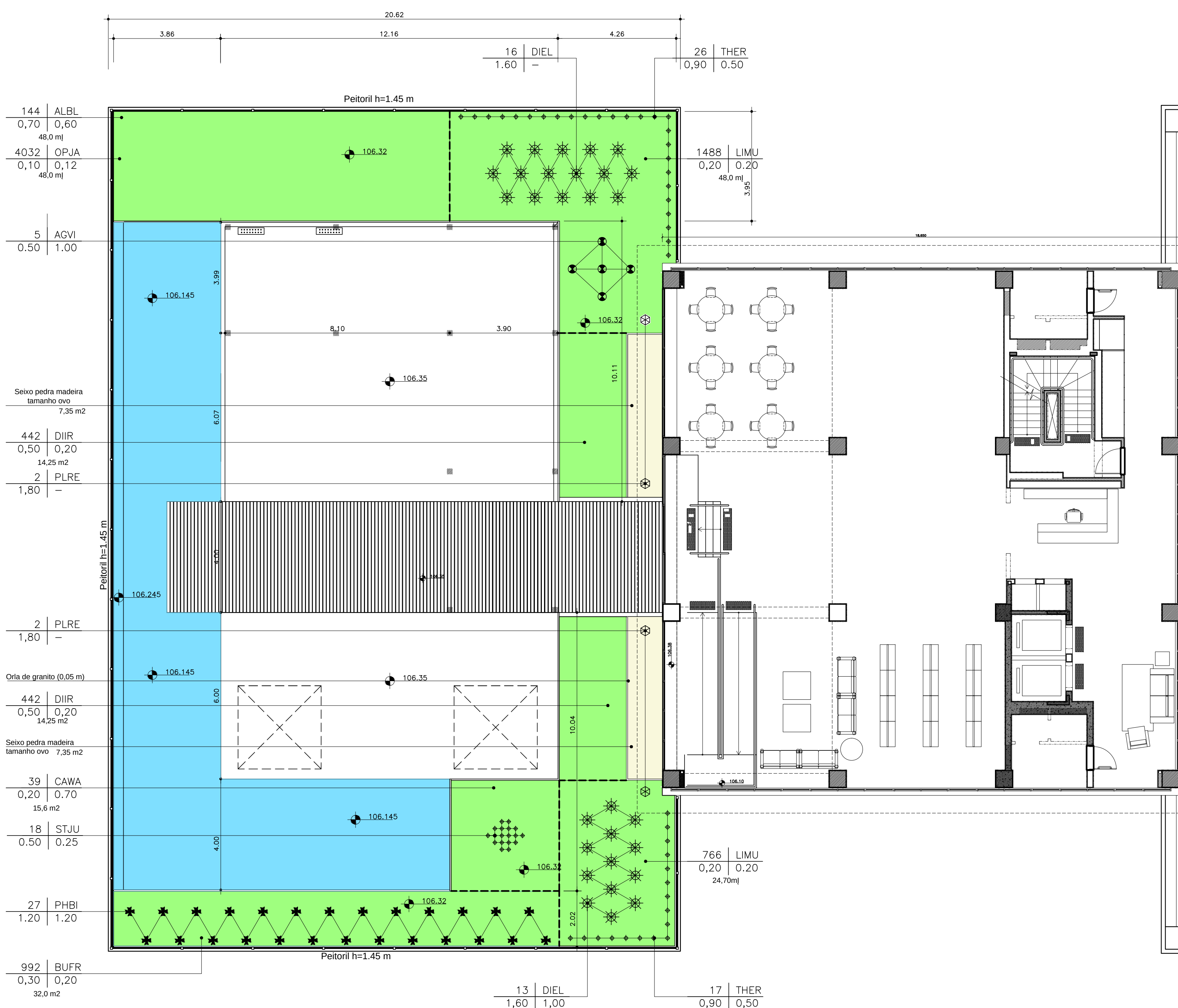
PLANTA - 10Jd sobre laje ESC 1:100
