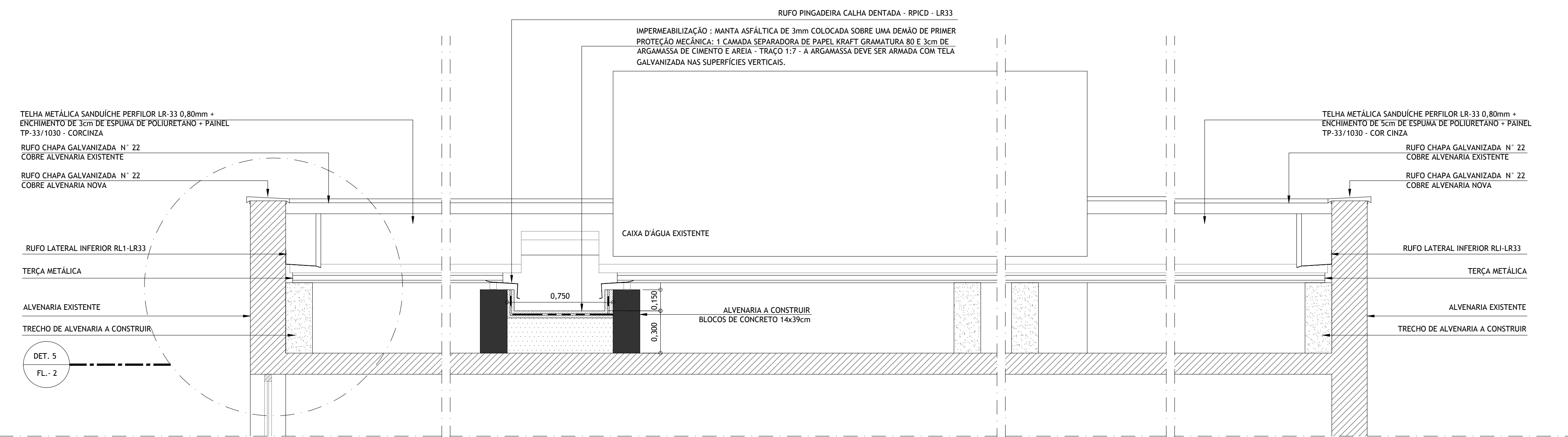
CORTE BB - TELHADO NOVO ESC.: 1:30 OBS.: O DIMENSIONAMENTO E DETALHES DOS PERFIS METÁLICOS ENCONTRAM-SE NO PROJETO DE ESTRUTURA
