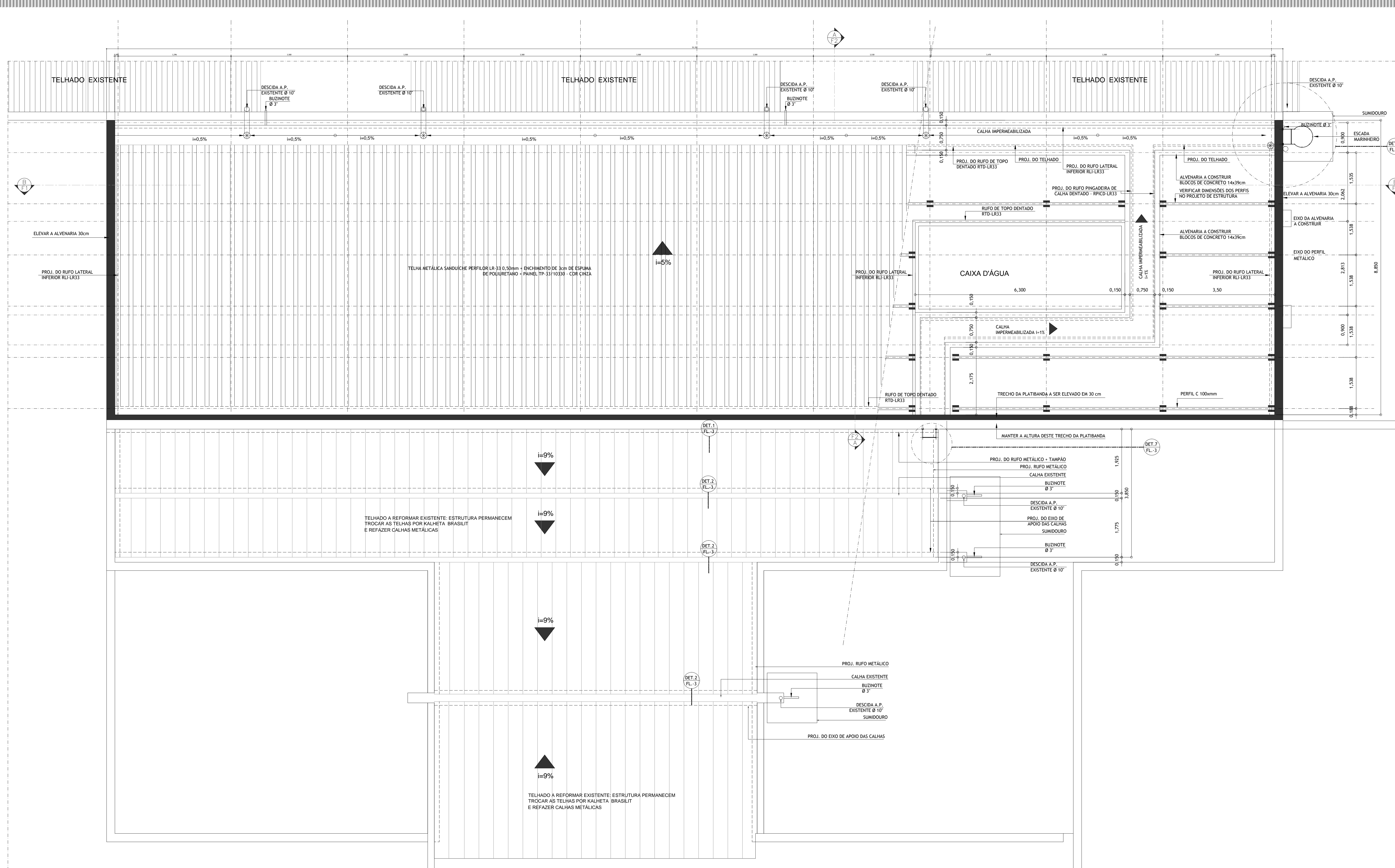
PLANTA DE COBERTURA - PARCIAL DOS TELHADOS A SEREM REFORMADOS E DO TELHADO NOVO ESC.: 1:30 OBS.: O DIMENSIONAMENTO E DETALHES DOS PERFIS METÁLICOS ENCONTRAM-SE NO PROJETO DE ESTRUTURA
