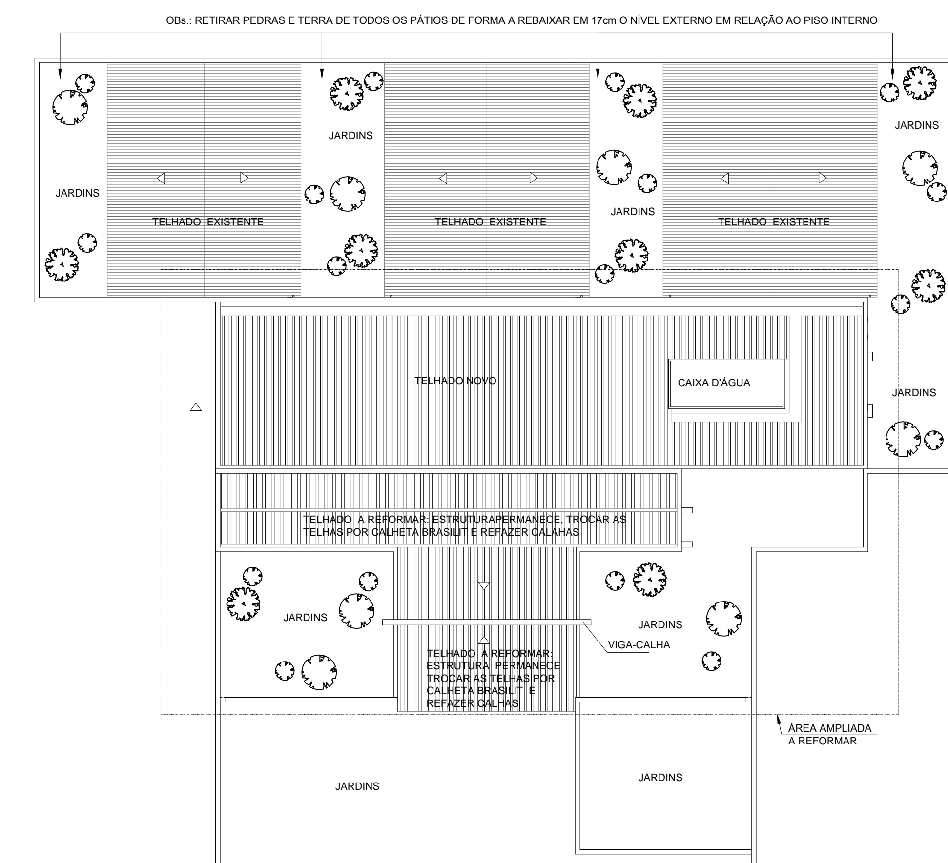
PLANTA DE SITUAÇÃO ESC.: 1:100
