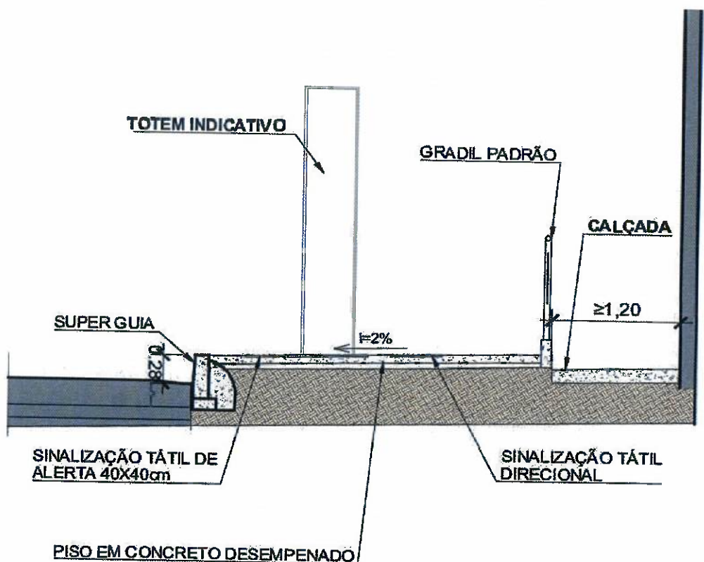
Figura 03: Seção transversal de parada com elevação parcial do passeio
