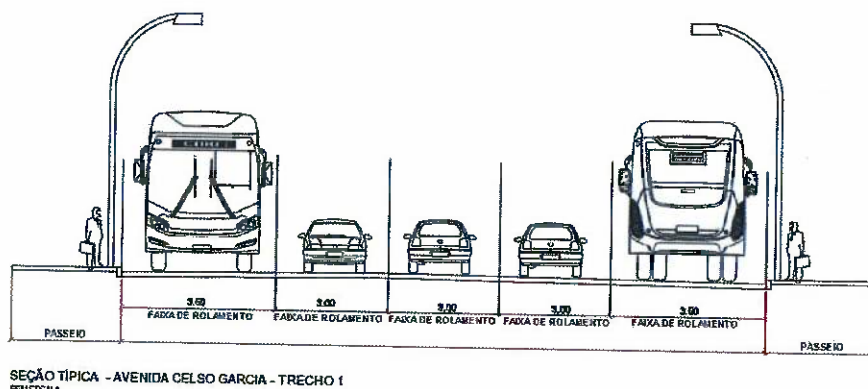
Figura 02: Seção típica da Requalificação da Av. Celso Garcia – Trecho 01
