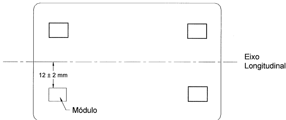
Figura 1 – Posicionamento do módulo eletrônico
