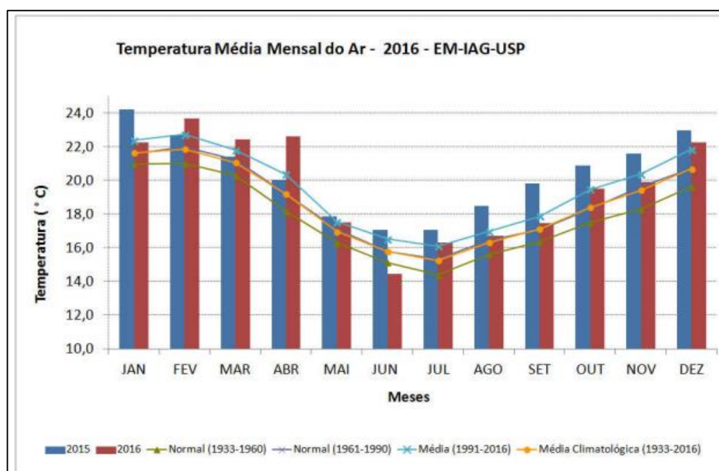
Figura 4: Temperaturas médias mensais do ar (2016) na Estação Meteorológica do Instituto de Astronomia, Geofísica e Ciências Atmosféricas da Universidade de São Paulo. Fonte: IAG/USP.
