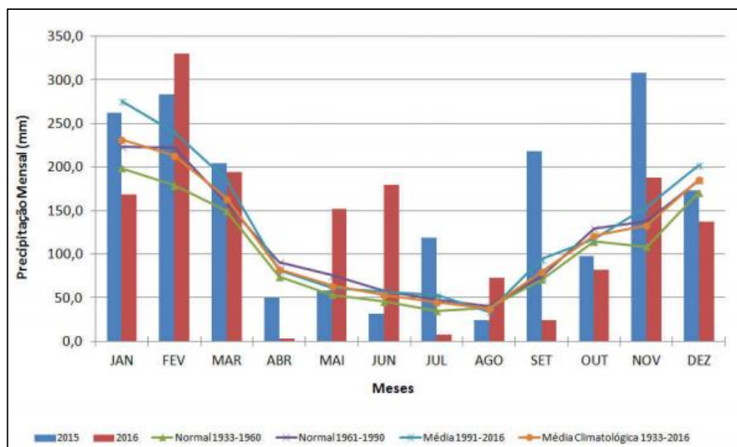
Figura 5: Precipitação mensal acumulada em São Paulo (SP) nos anos de 2015 e 2016, além das normais e da média climatológica. Fonte: IAG/USP.
