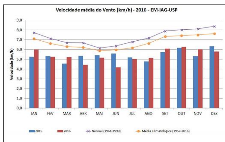
Figura 6: Velocidade média mensal do vento (km/h) nos anos de 2015 e 2016, além da normal e da média climatológica. Fonte: IAG.
