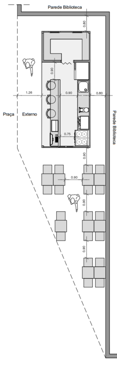
Figura 10 – Planta Baixa: ESPAÇO GASTRONÔMICO
