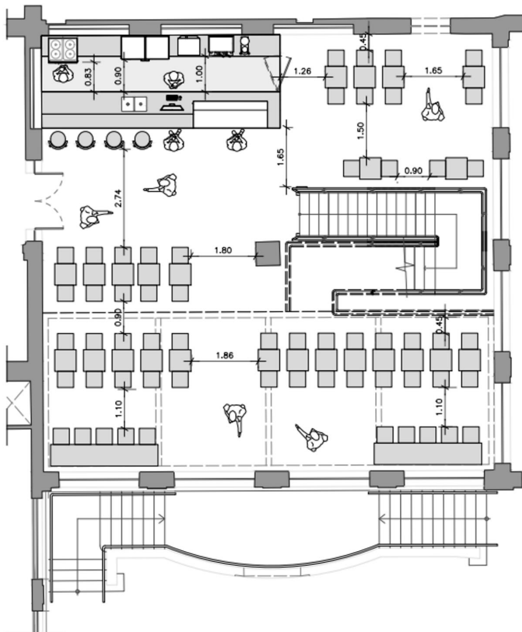
PLANTA BAIXA – ESPAÇO GASTRONÔMICO Sem Escala
