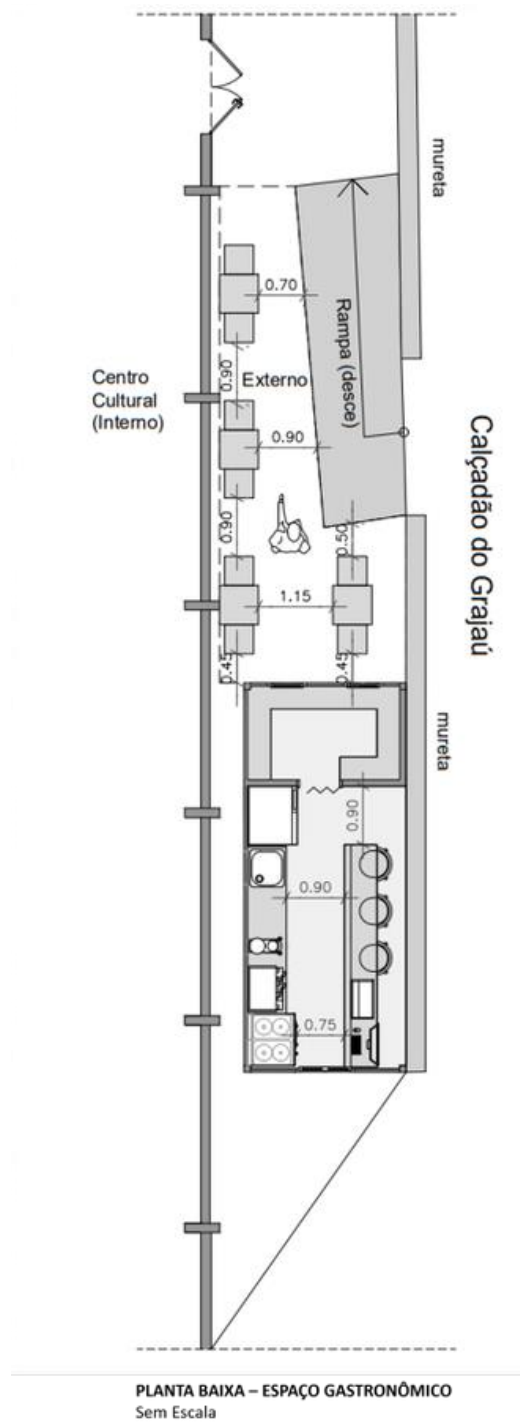
Figura 12 – Planta Baixa: Espaço Gastronomico
