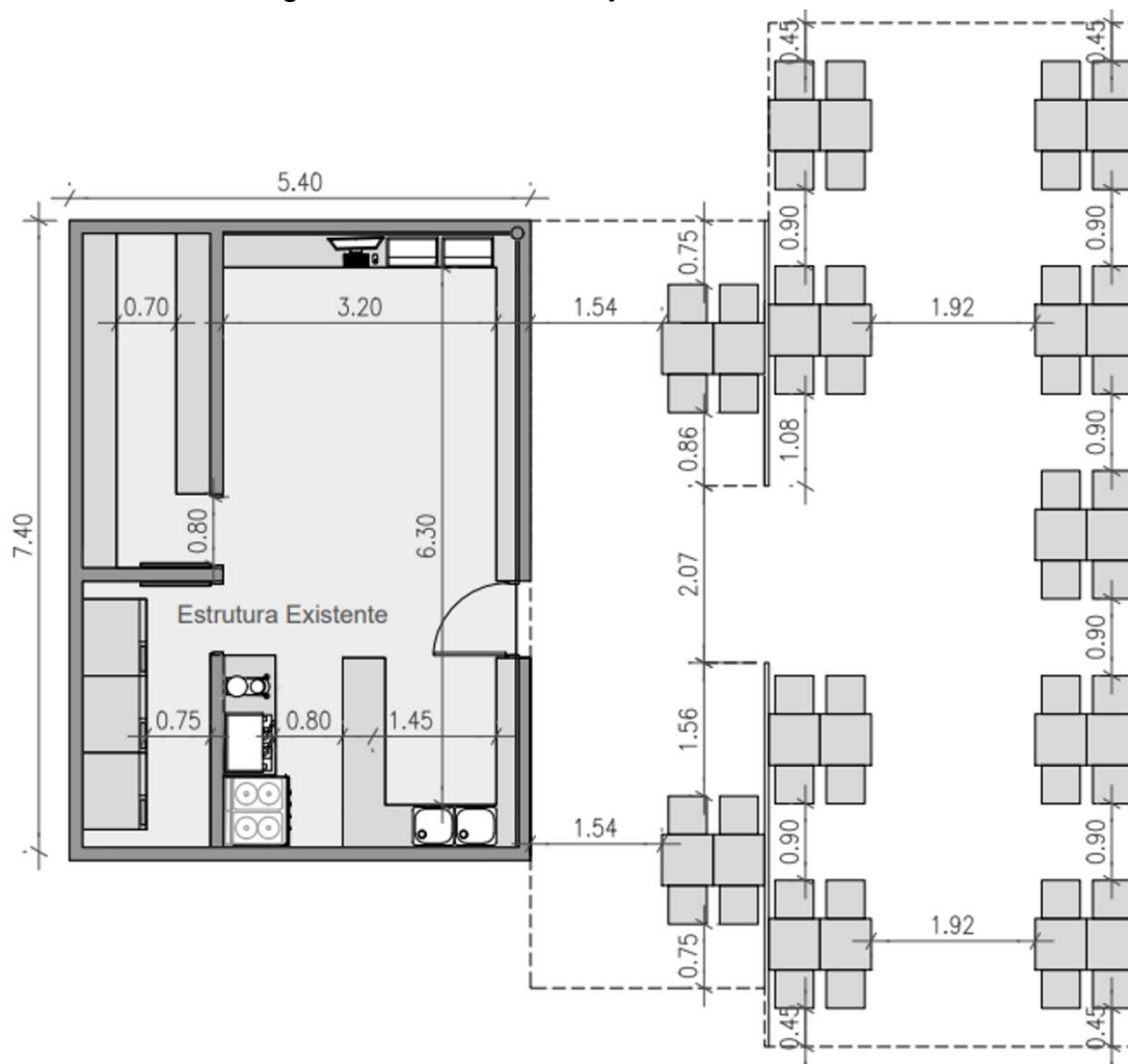
PLANTA BAIXA – ESPAÇO GASTRONÔMICO
