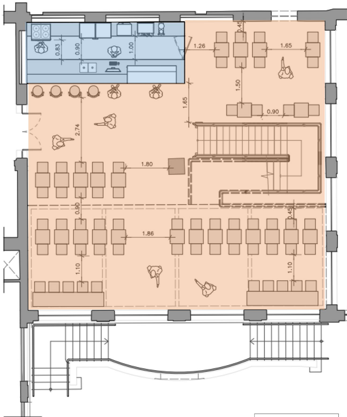
Figura 2 – Planta da ÁREA DA PERMISSÃO 21
