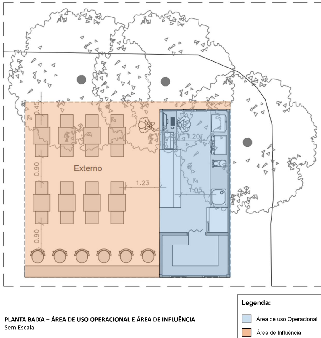
Figura 2 – Planta da ÁREA DA PERMISSÃO 20
