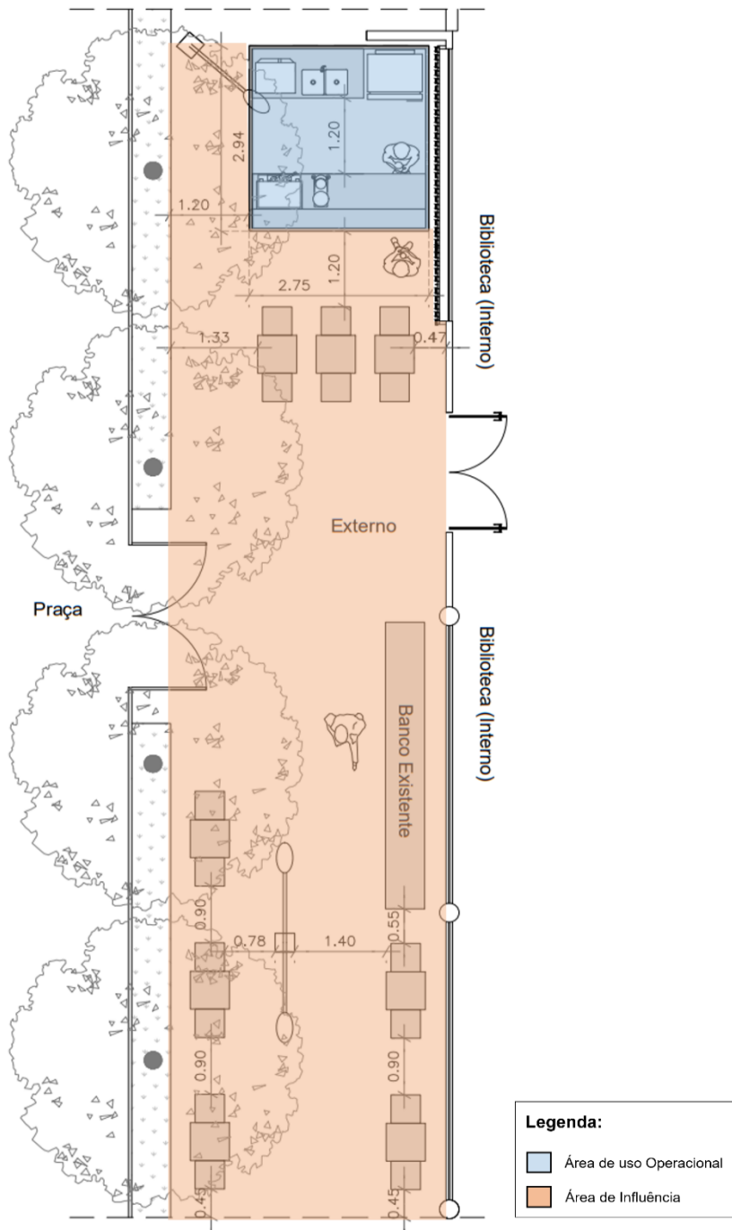
PLANTA BAIXA – ÁREA DE USO OPERACIONAL E ÁREA DE INFLUÊNCIA Sem Escala
