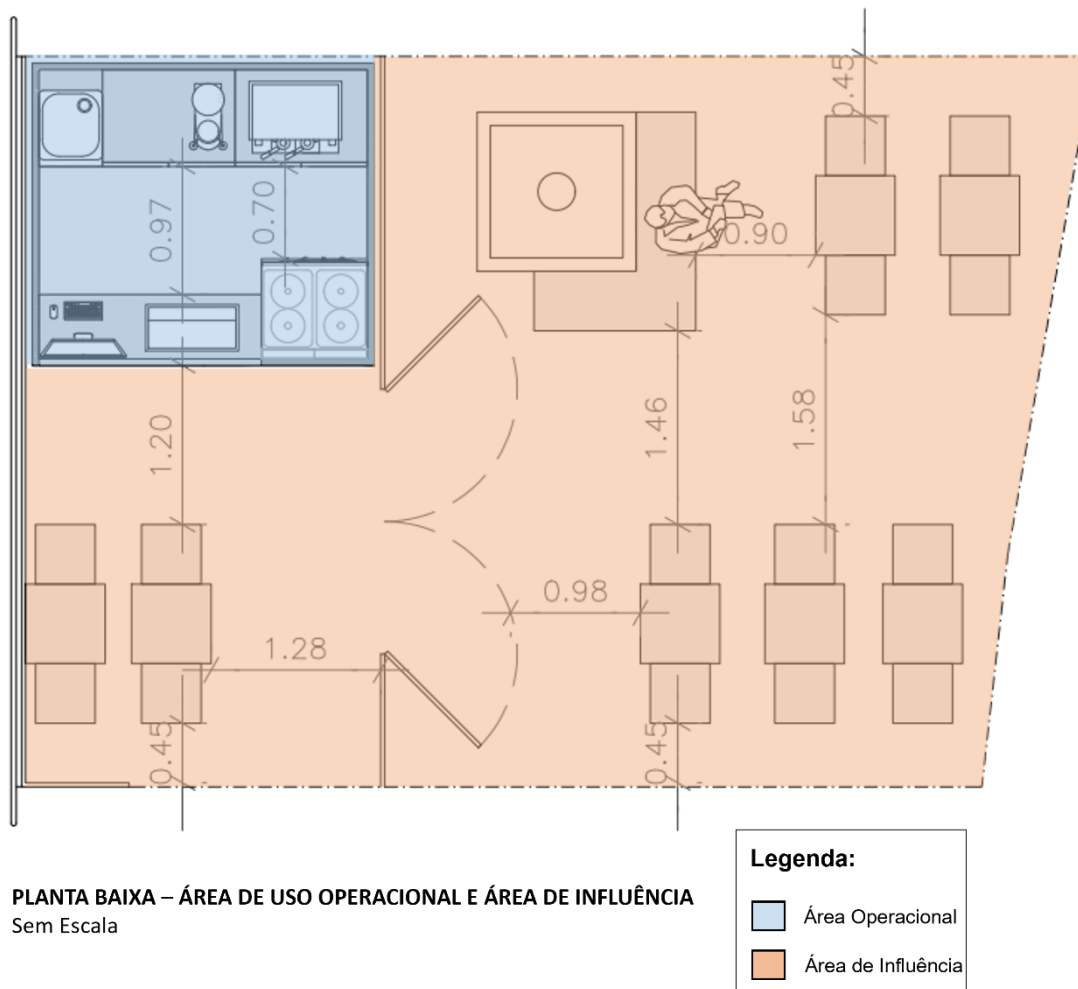
Figura 2 - Planta da ÁREA DA PERMISSÃO 1
