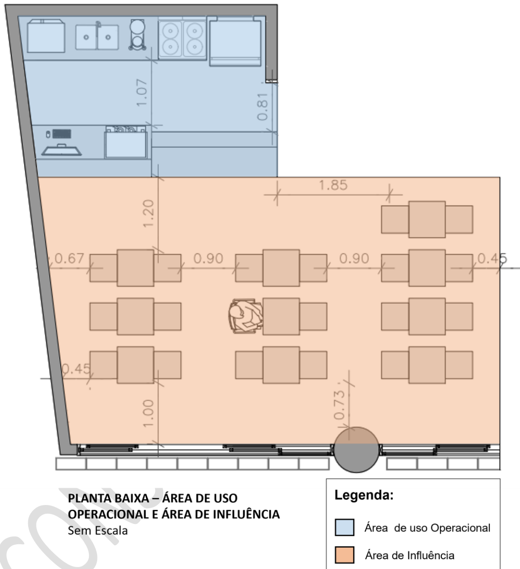
Figura 10– Planta Baixa Térreo: ÁREA DE USO OPERACIONAL e ÁREA DE INFLUÊNCIA
