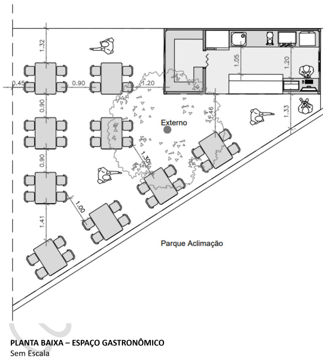
Figura 12 – Planta Baixa: ESPAÇO GASTRONÔMICO
