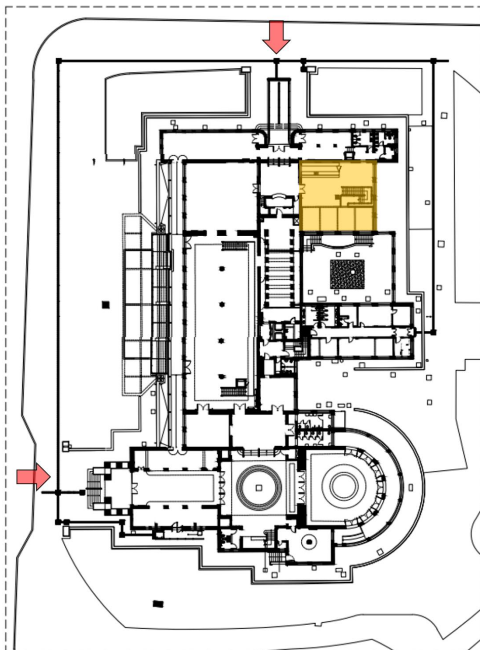
Figura 8 – Planta Baixa: Térreo
