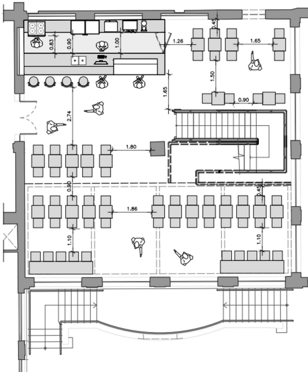
Figura 10 – Planta Baixa: ESPAÇO GASTRONÔMICO
