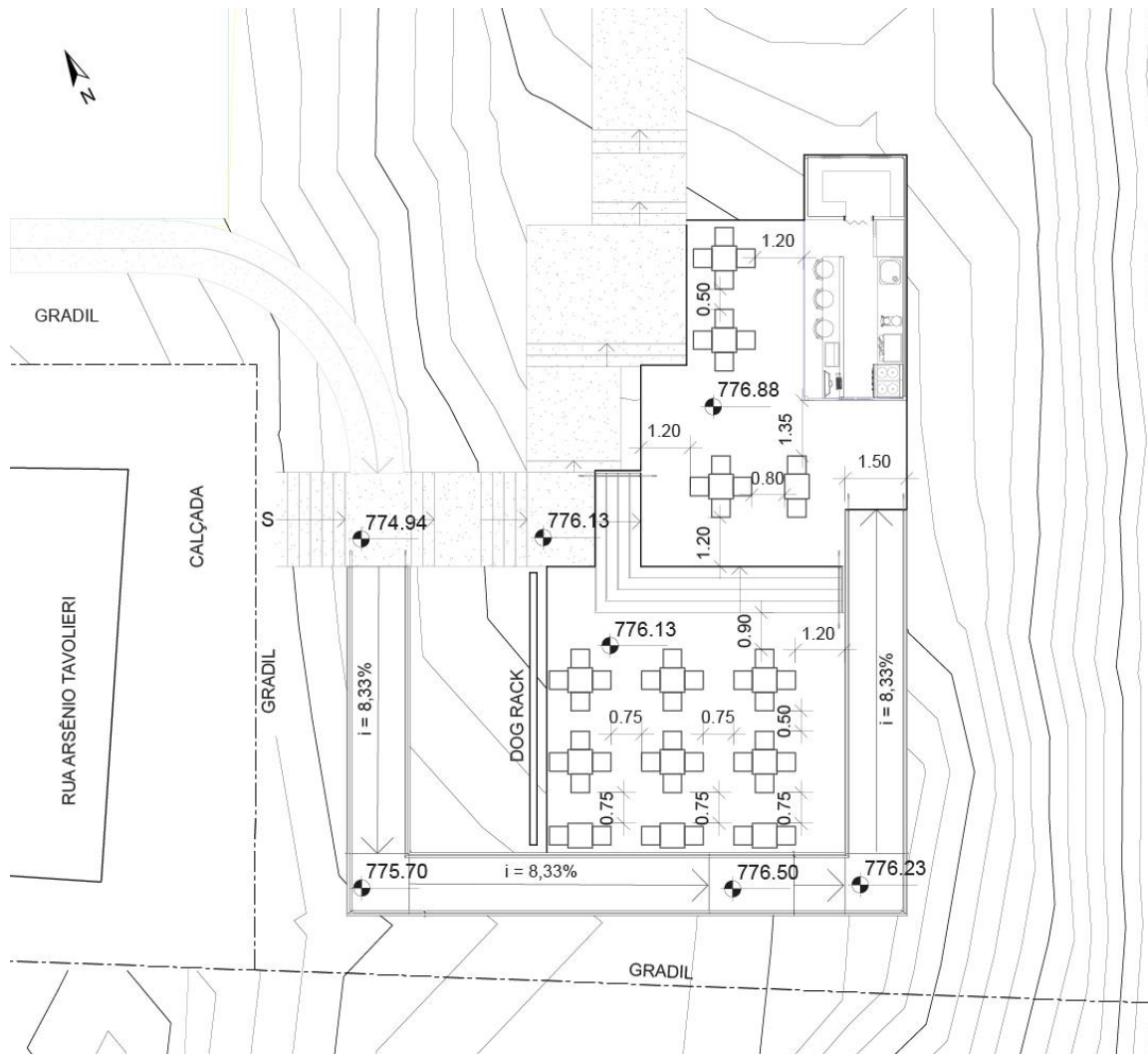
Figura 10 – Planta Baixa: ESPAÇO GASTRONÔMICO
