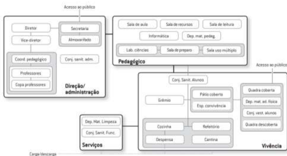
Figura 3. Organização dos ambientes do BLOCO EMEF.
