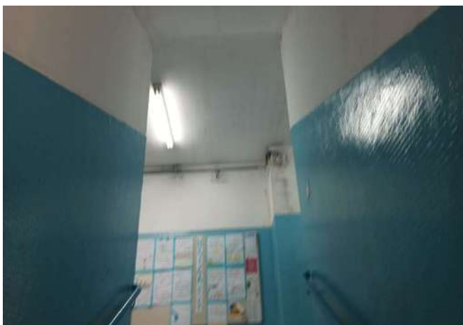
FOTO 149 ESCADARIA SEM CORRIMÃO CONTÍNUO
