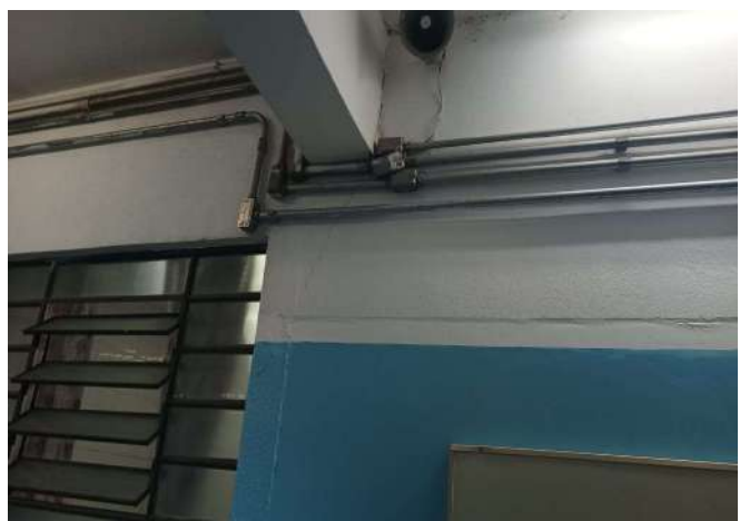
FOTO 208 CORREDORES COM AUSÊNCIA DE JUNTA DE DILATAÇÃO
