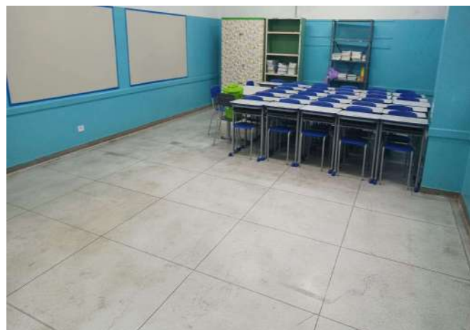
FOTO 252 SALA DE AULA 18 COM FISSURA NO PISO
