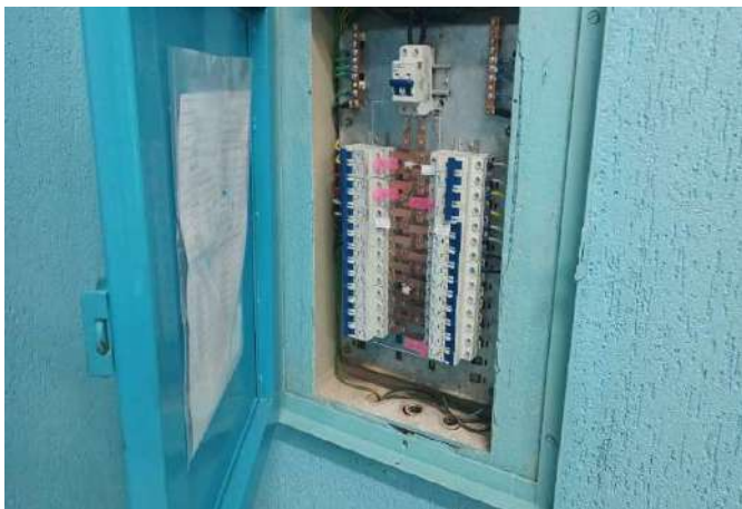
FOTO 241 QUADRO DE DISTRIBUIÇÃO DE LUZ
