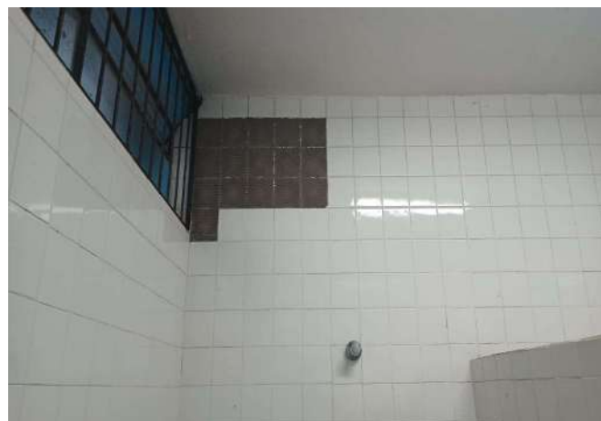
FOTO 120 BANHEIRO FEMININO DE ALUNOS COM DESTACAMENTO DOS REVESTIMENTOS
