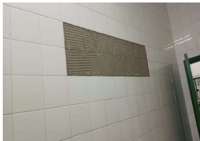
FOTO 28 BANHEIRO DE FUNCIONÁRIOS FEMININO COM DESTACAMENTO DOS REVESTIMENTOS
