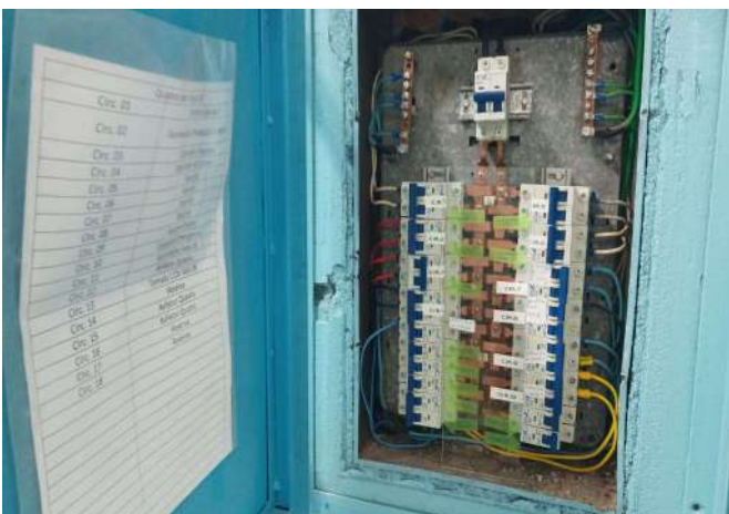
FOTO 162 QUADRO DE DISTRIBUIÇÃO DE LUZ
