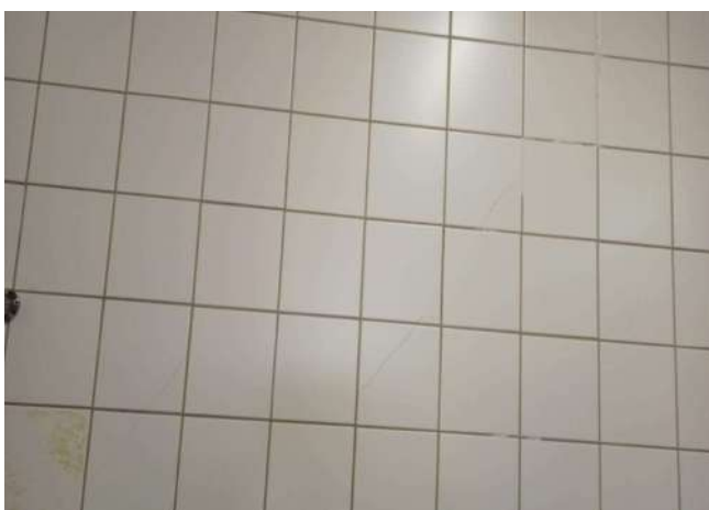
FOTO 93 COZINHA / PAREDE COM TRINCAS
