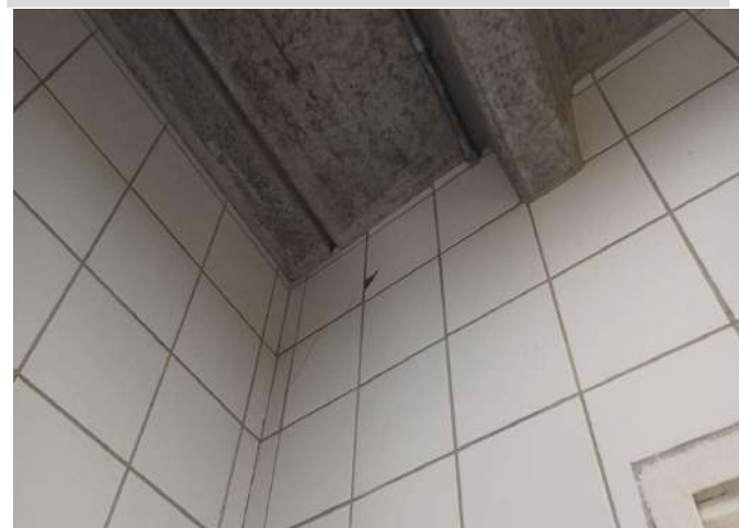
FOTO 213 BANHEIRO FEM ALUNO / REVESTIMENTO DANIFICADO
