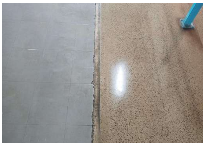
FOTO 106 PÁTIO COBERTO / PISO SEM JUNTA DE DILATAÇÃO.
