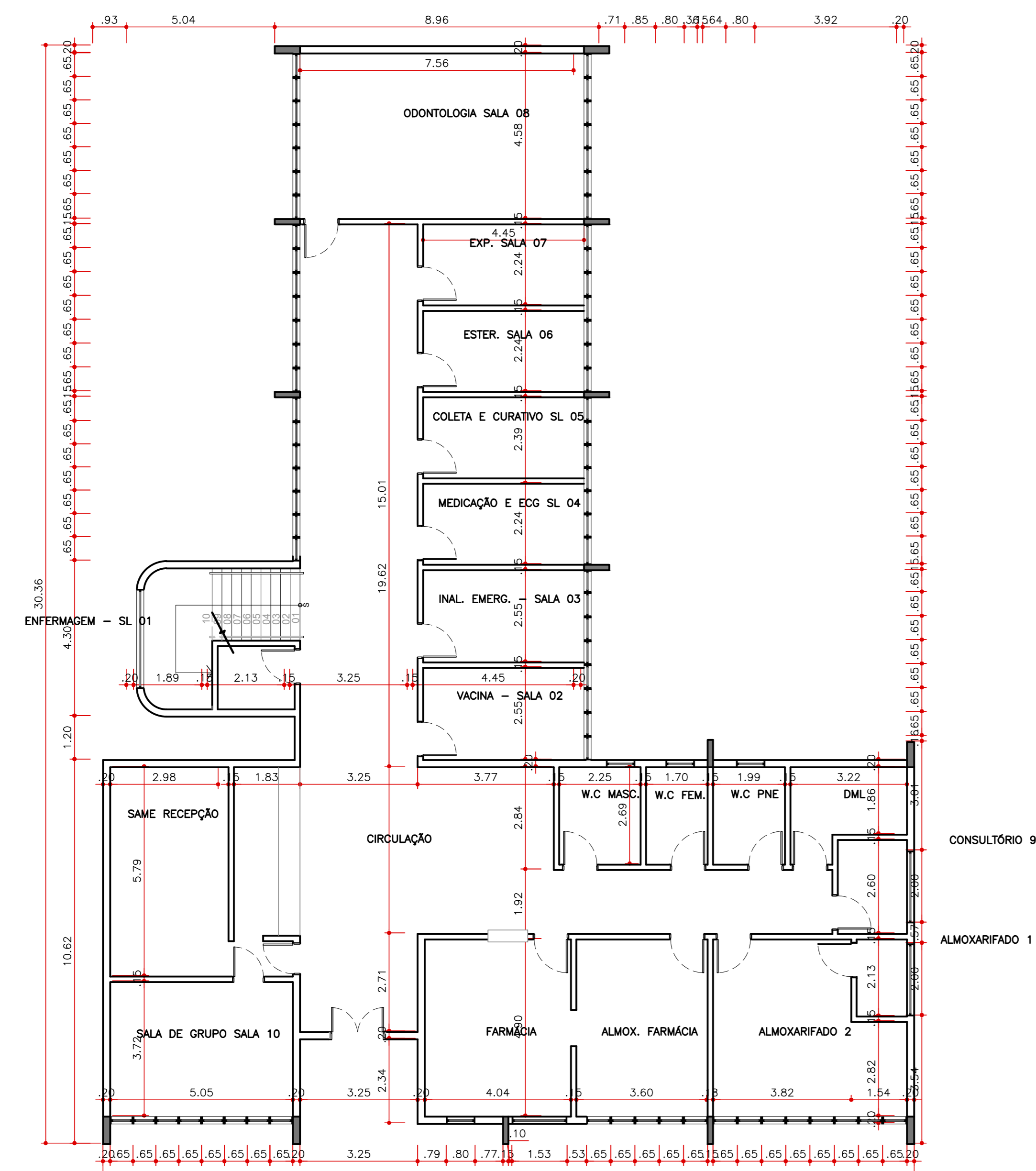
PLANTA DE DIMENSIONAMENTO - TÉRREO UBS VILA BORGES ESCALA: 1:100
