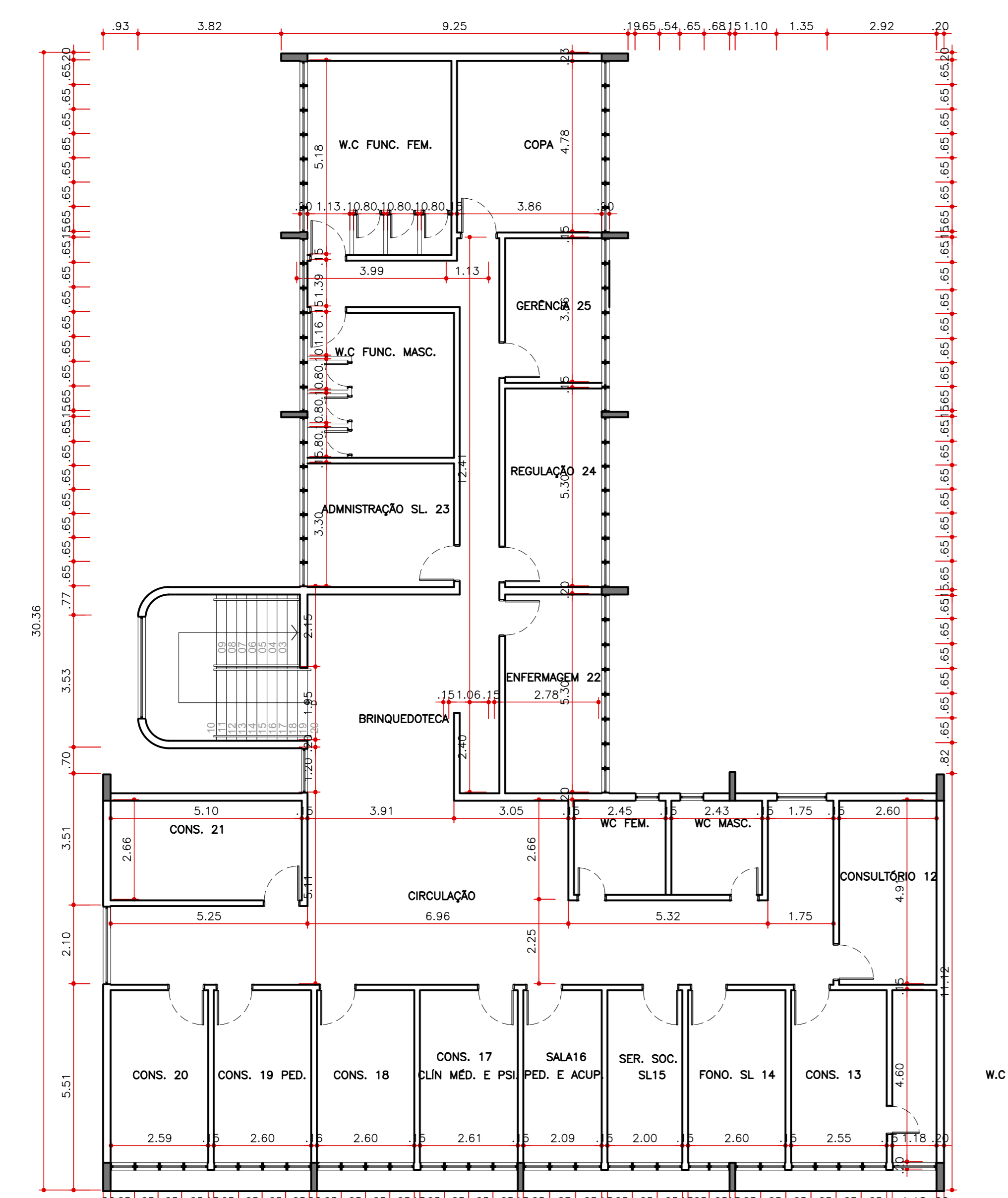
PLANTA DE DIMENSIONAMENTO - 1º PAVIMENTO UBS VILA BORGES ESCALA: 1:100
