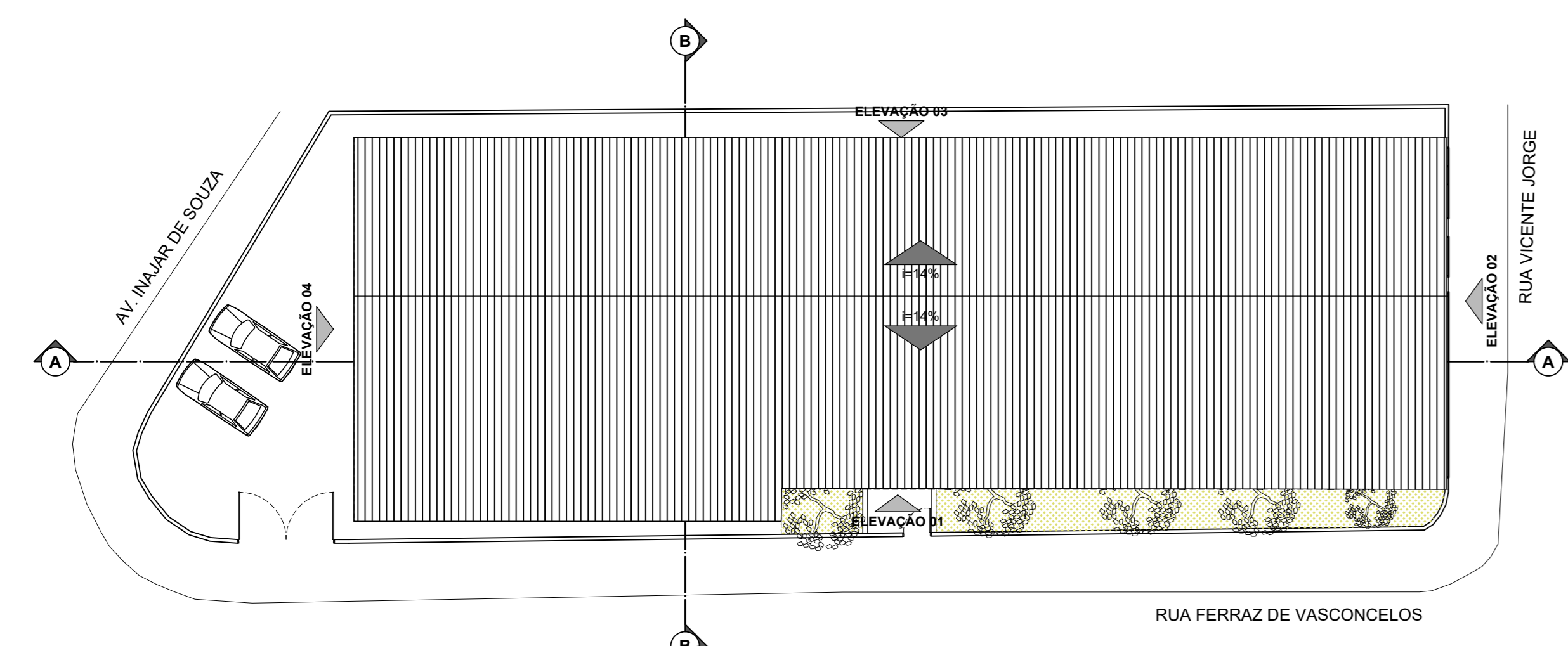
IMPLANTAÇÃO E COBERTURA UBS VILA RAMOS FREGUESIA DO Ó ESCALA: 1:200
