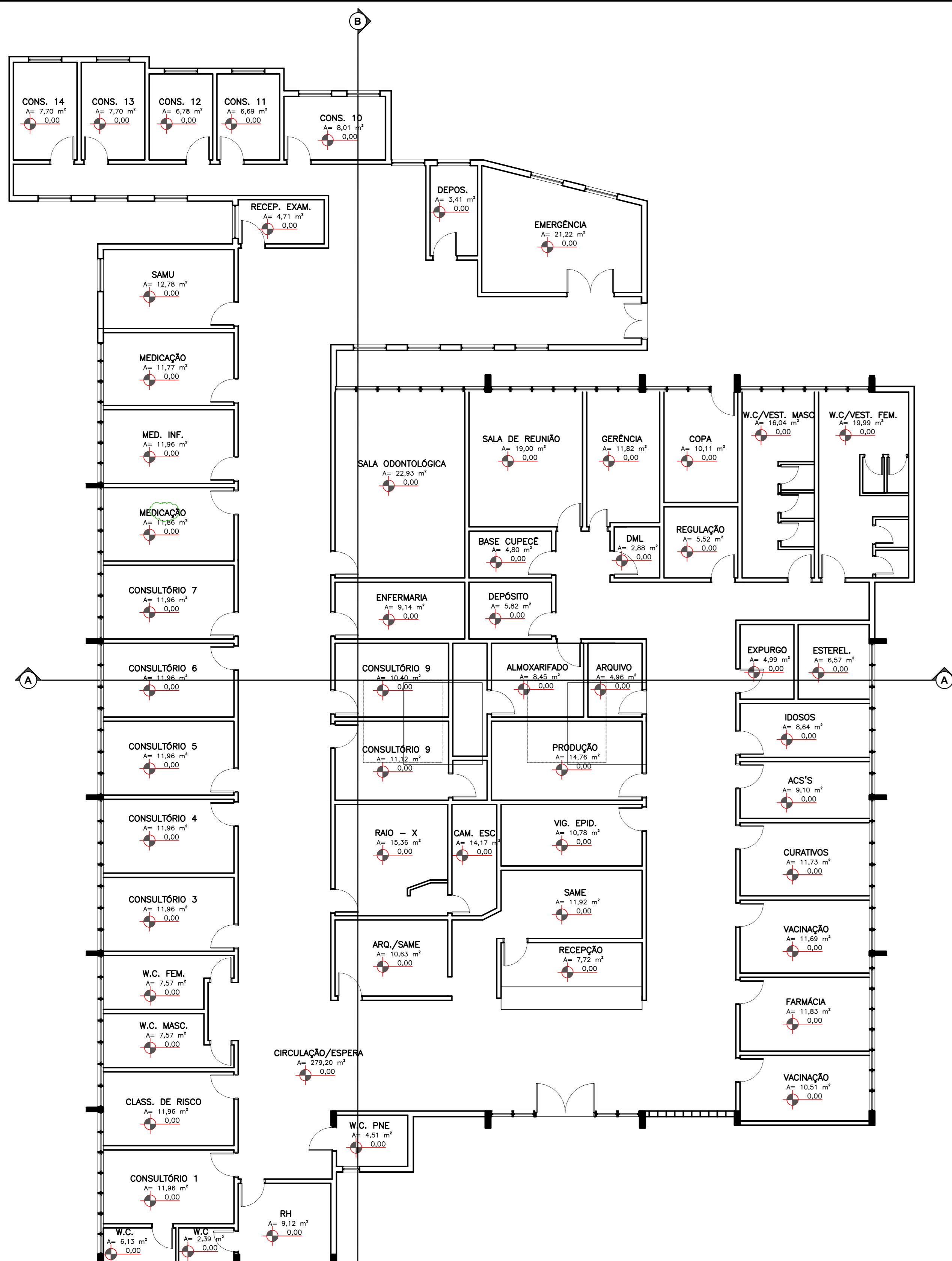
PLANTA DE LAYOUT UBS CUPECÉ - WALDEMIRO PREGNOLATTO ESCALA: 1:100
