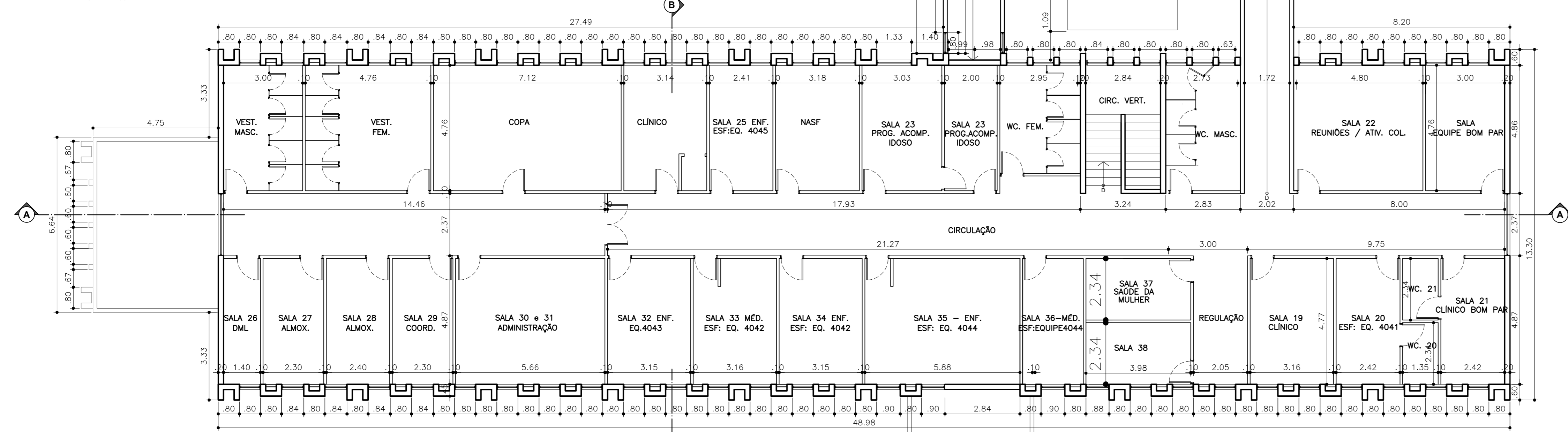
DIMENSIONAMENTO - 1º PAVIMENTO UBS/AMA - PARI ESCALA: 1:100
