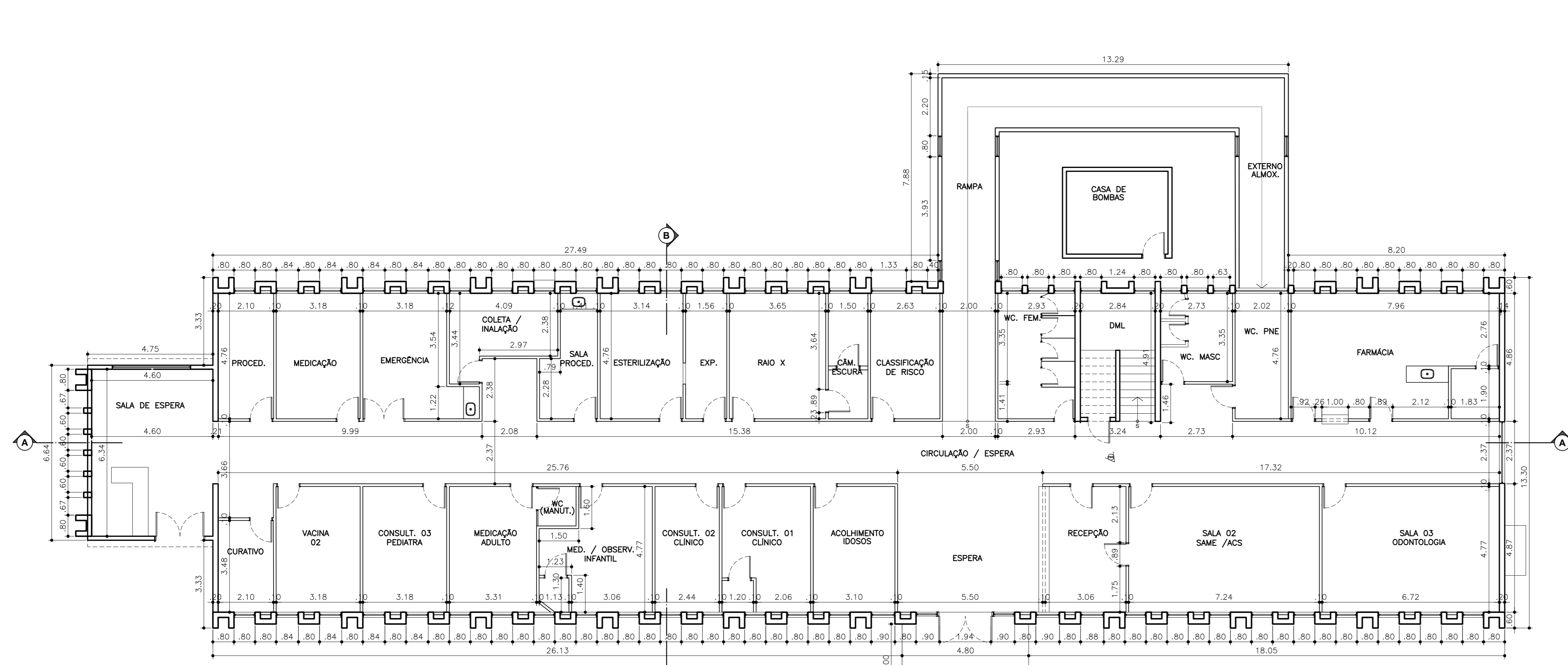
DIMENSIONAMENTO - TERREO UBS/AMA - PARI ESCALA: 1:100
