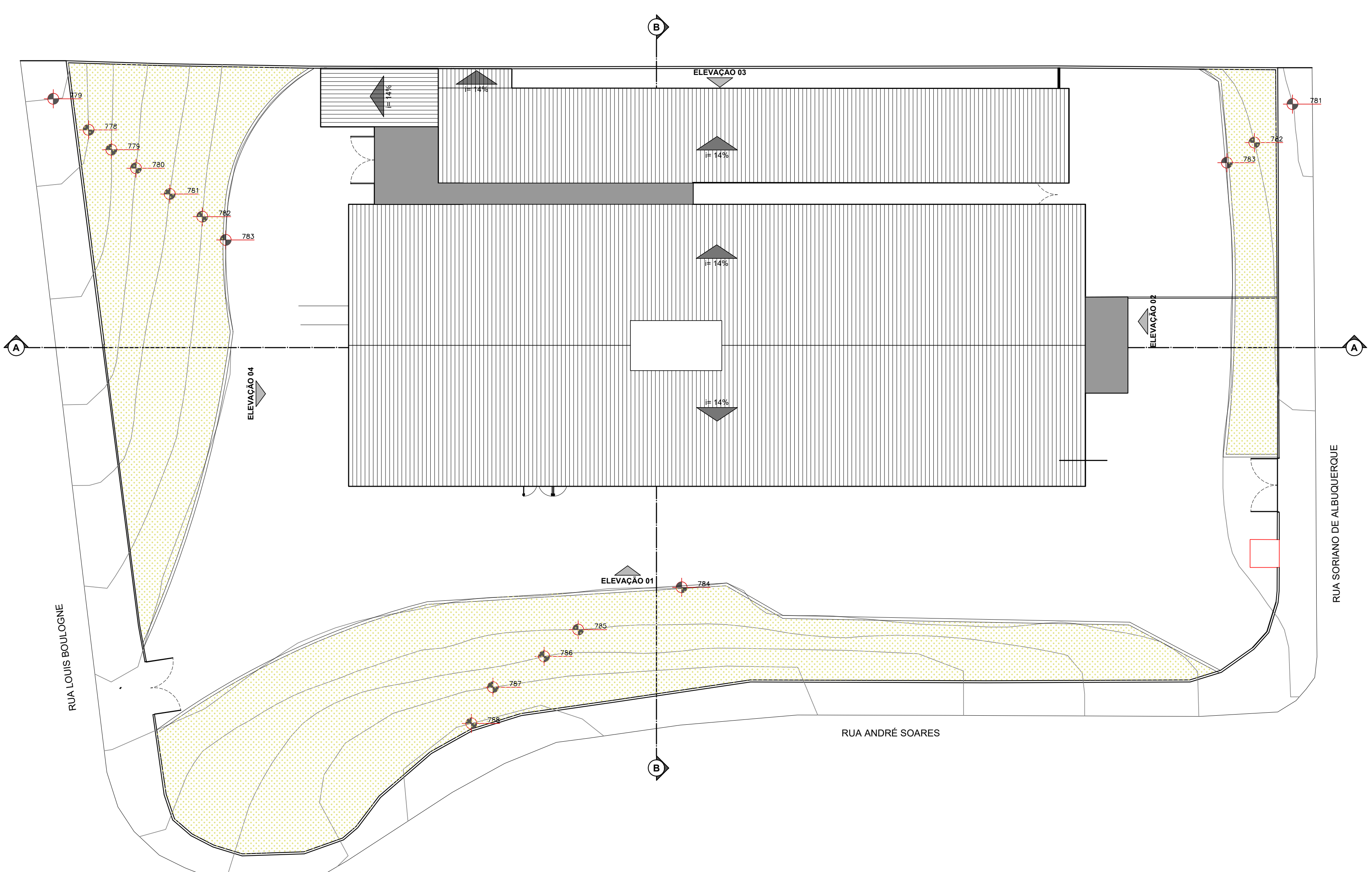
IMPLANTÇÃO E COBERTURA UBS PA JARDIM MACEDÔNIA ESCALA: 1/200
