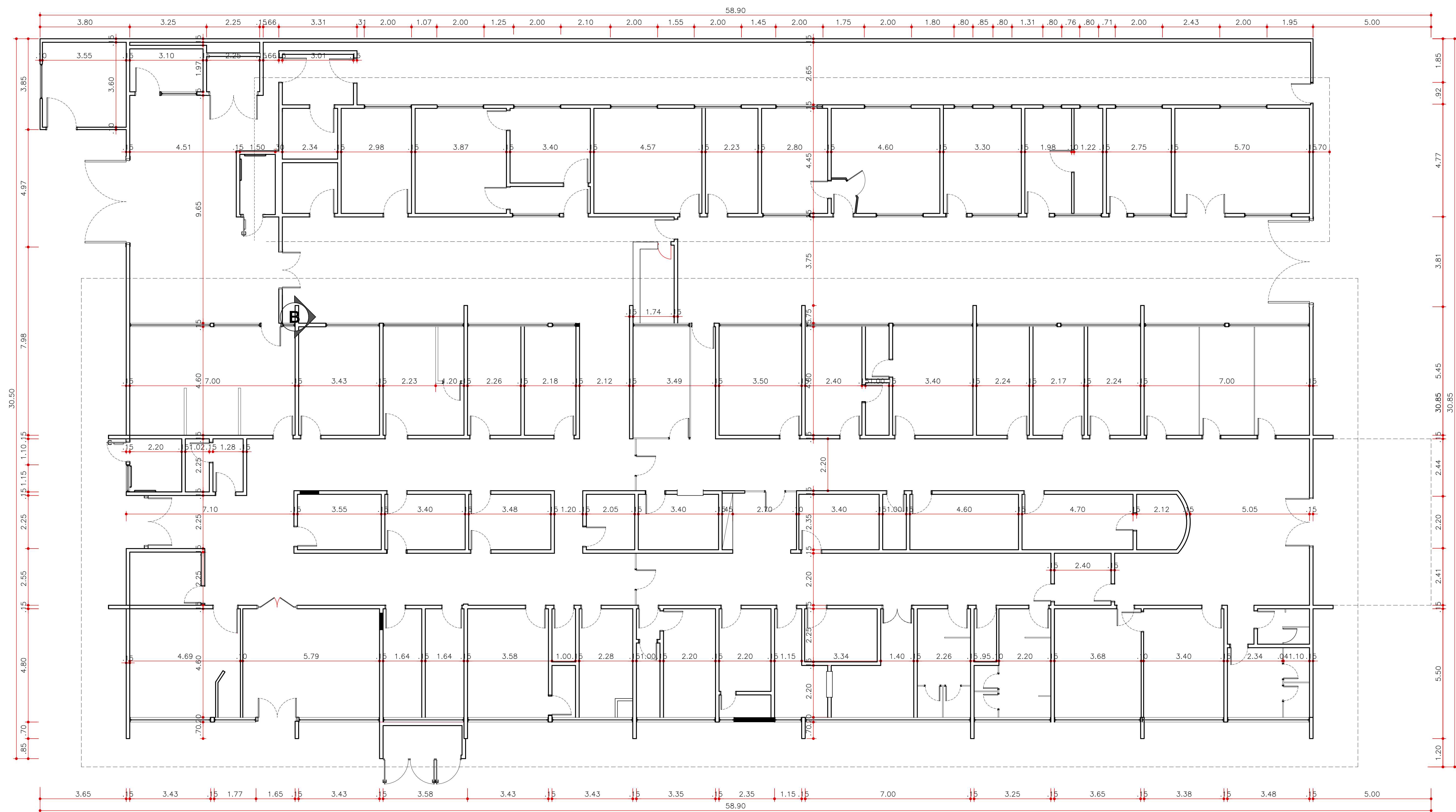
DIMENSIONAMENTO UBS PA JARDIM MACEDÔNIA ESCALA: 1/75
