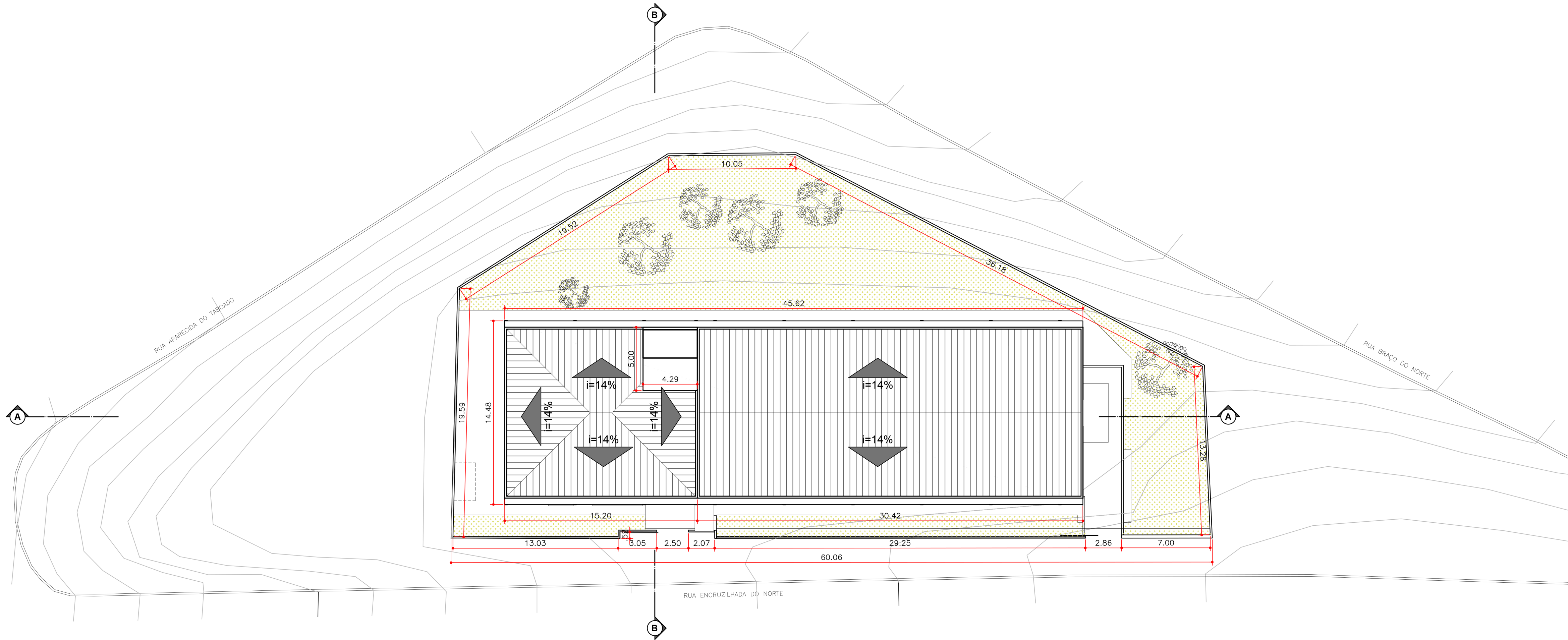
IMPLANTAÇÃO E COBERTURA AMA / UBS JARDIM PAULISTANO ESCALA: 1:200
