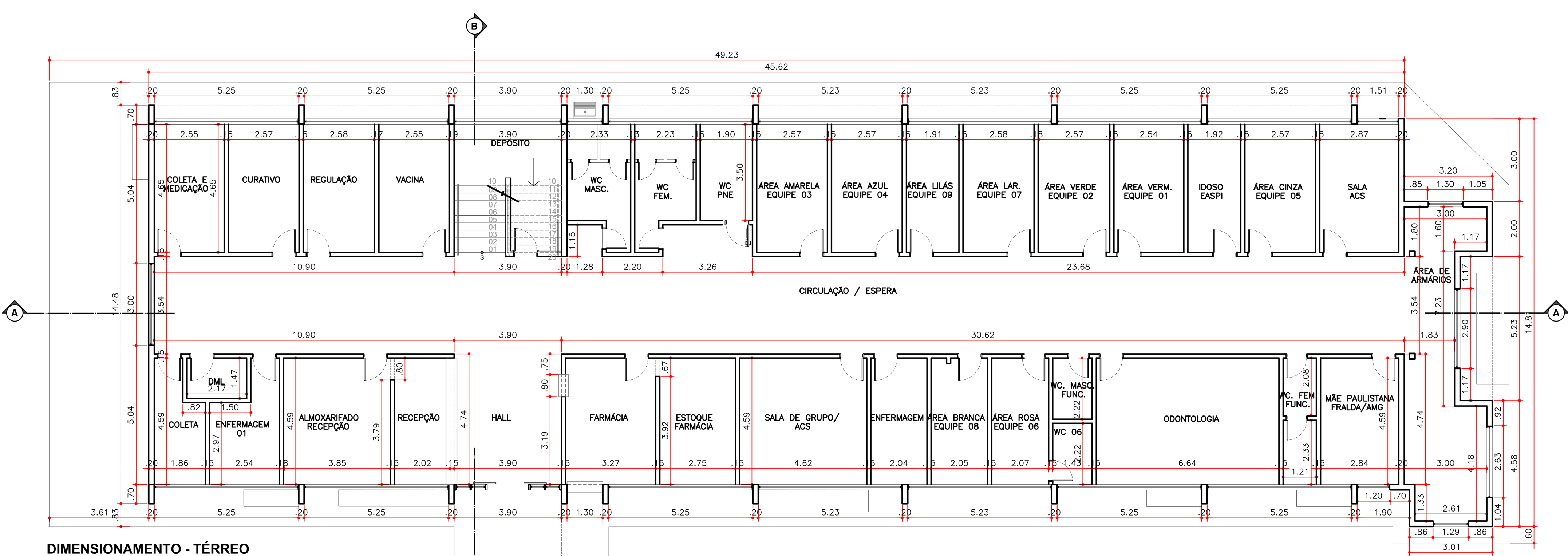
DIMENSIONAMENTO - TÉRREO AMA / UBS JARDIM PAULISTANO ESCALA: 1:100
