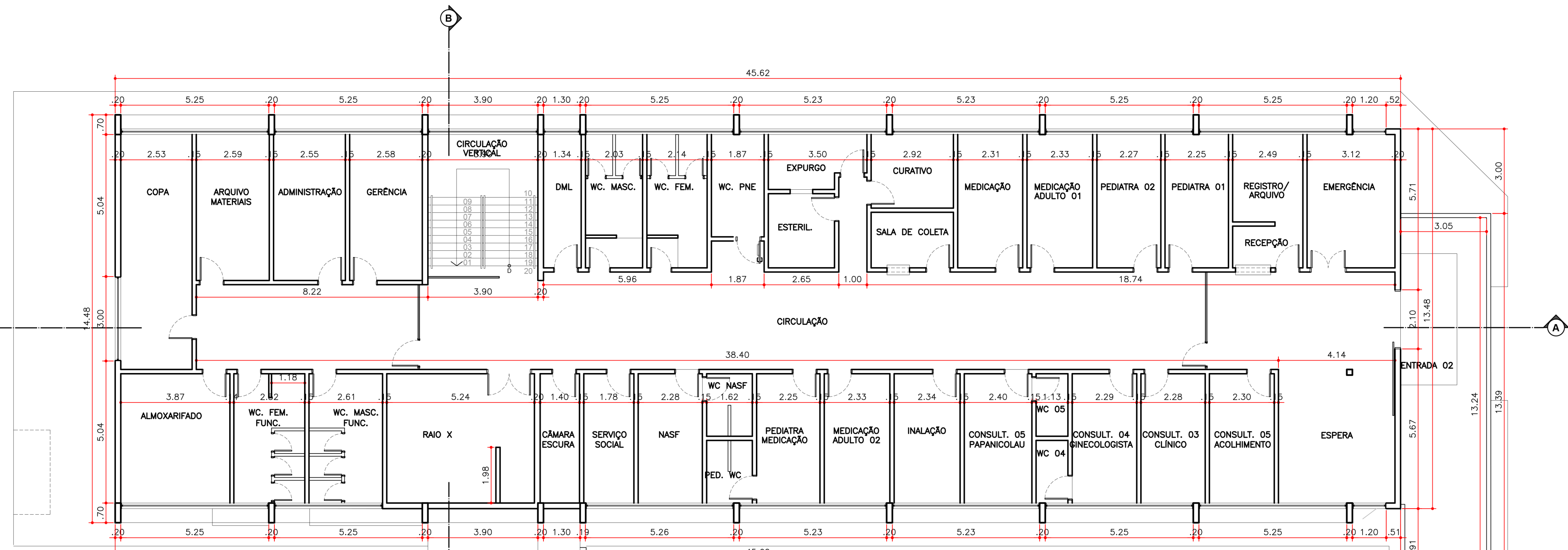
DIMENSIONAMENTO - 1º PAVIMENTO AMA / UBS JARDIM PAULISTANO ESCALA: 1:100
