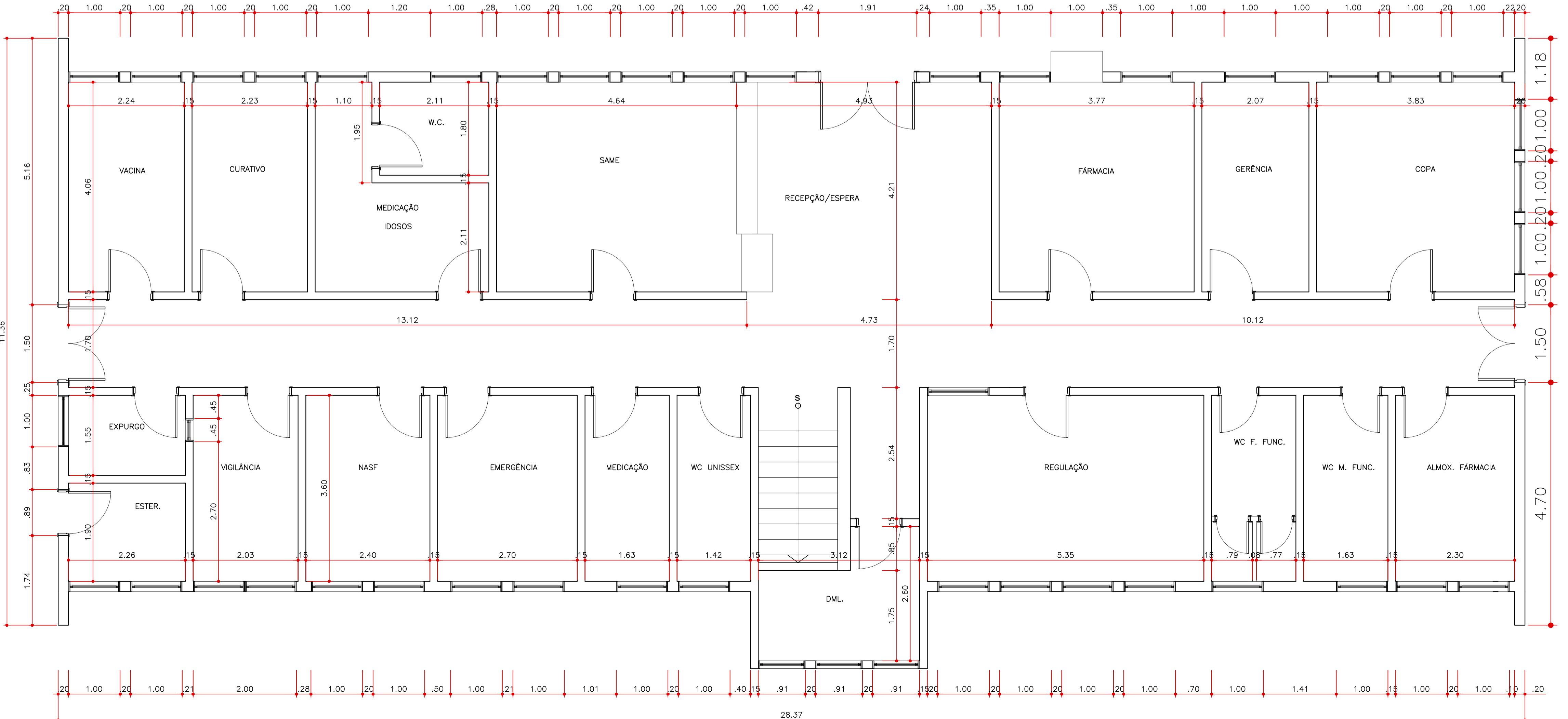
DIMENSIONAMENTO - TÉRREO UBS JARDIM D'ABRIL ESCALA:1:50
