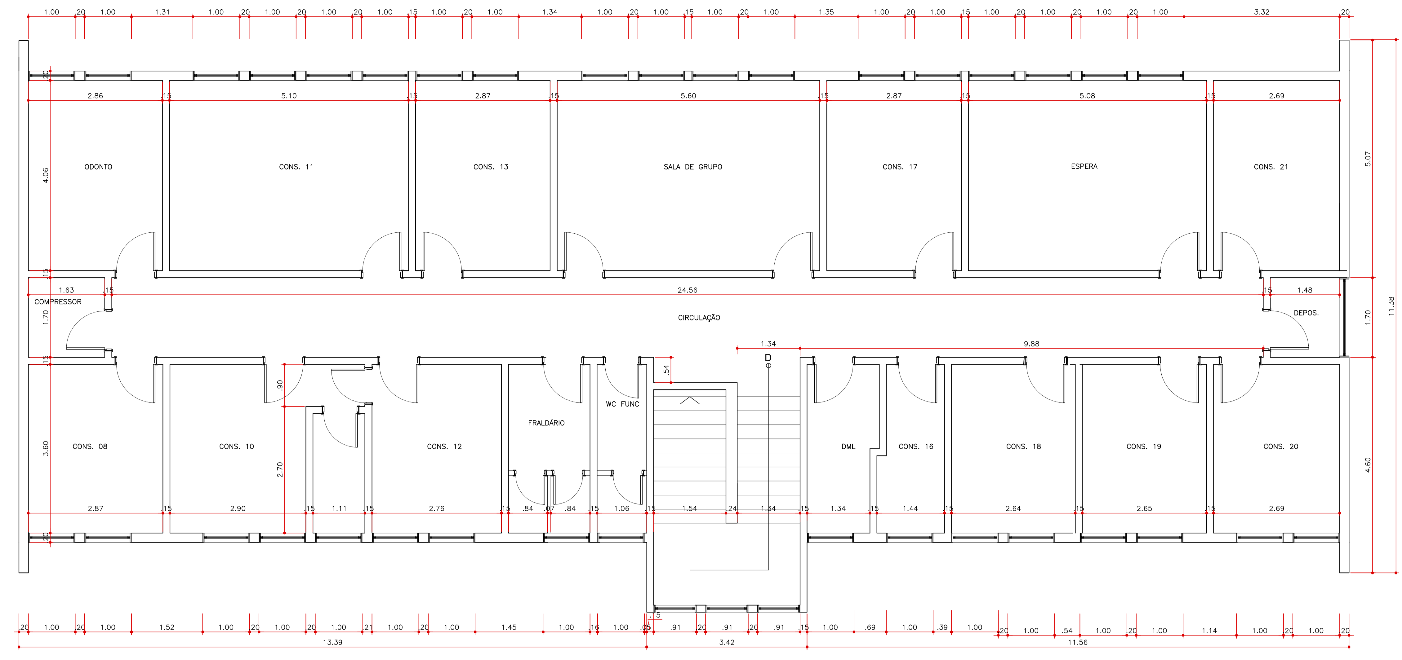
DIMENSIONAMENTO - 1º PAVIMENTO UBS JARDIM D'ABRIL ESCALA:1:50
