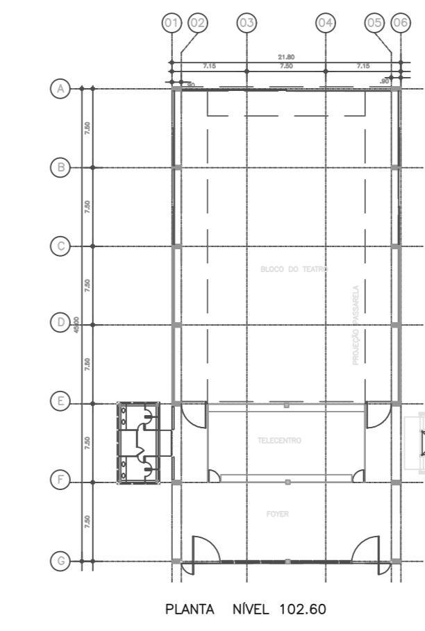
TÉRREO
