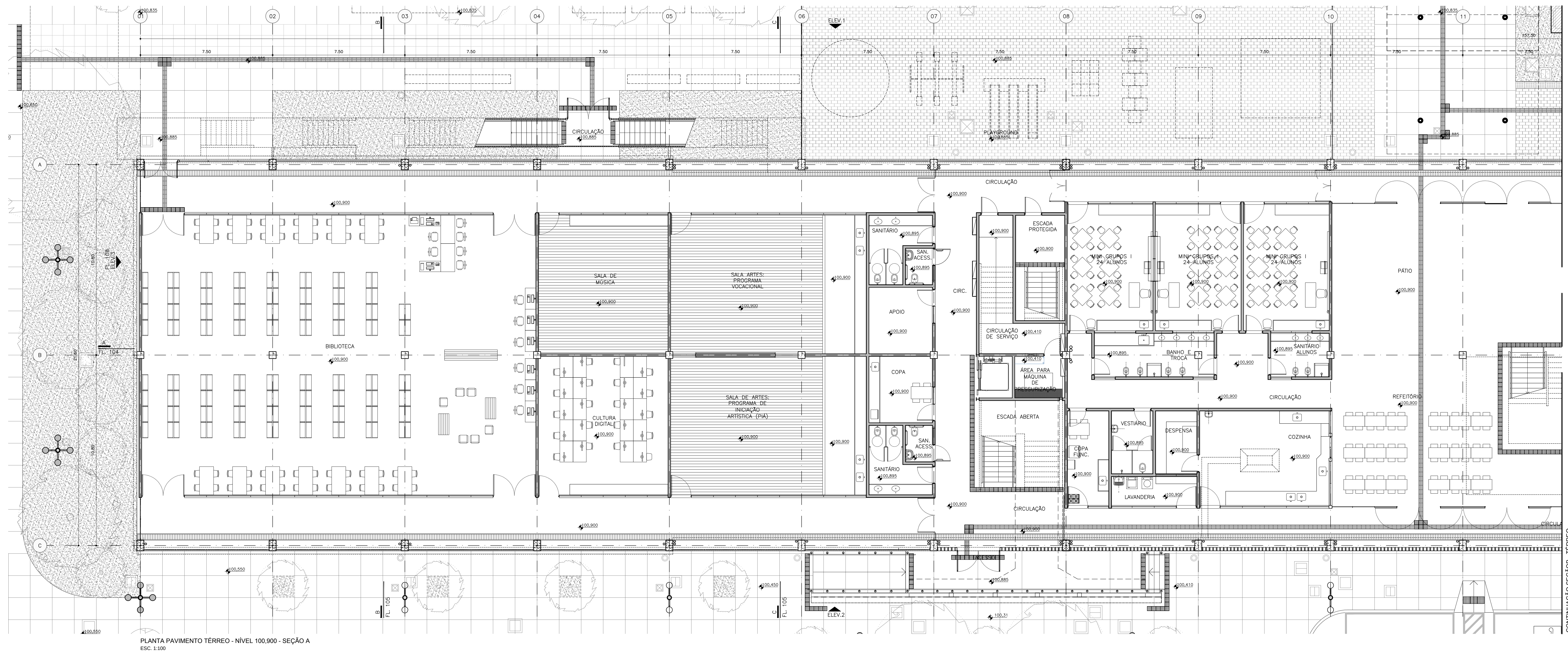
PLANTA PAVIMENTO TÉRREO - NÍVEL 100.900 - SEÇÃO A ESC. 1:100
