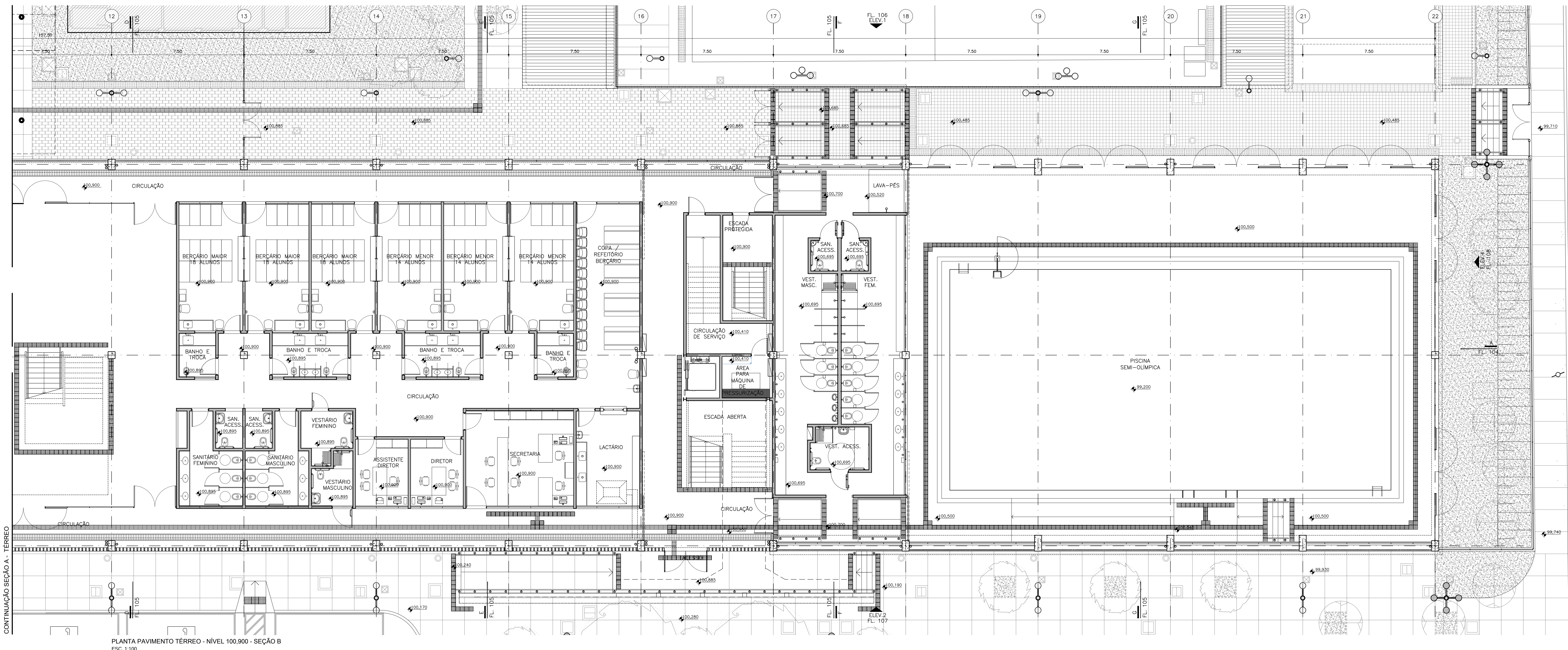
PLANTA PAVIMENTO TÉRREO - NÍVEL 100.900 - SEÇÃO B ESC. 1:100
