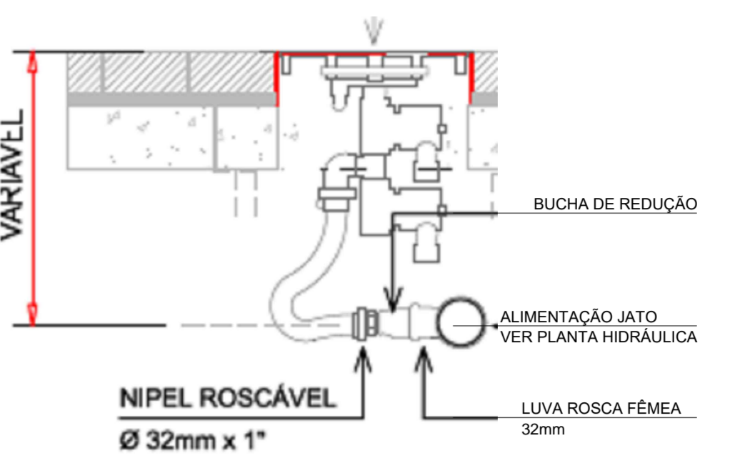
DETALHE DE MONTAGEM SEM ESCALA
