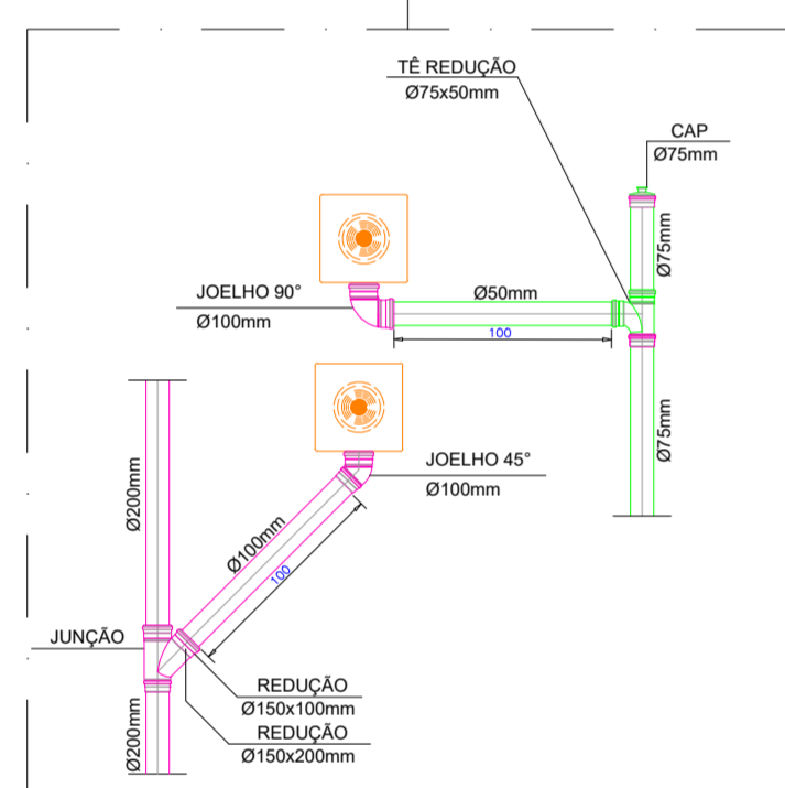
DETALHE "C" JATOS NEVOA SEM ESCALA
