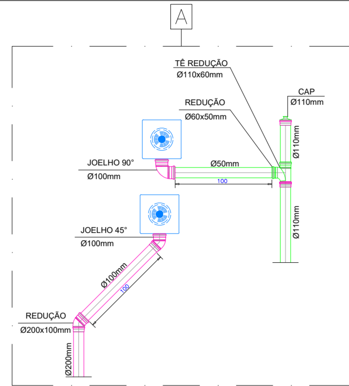
DETALHE "A" JATOS VERTICAIS SEM ESCALA
