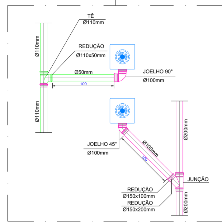
DETALHE "B" JATOS VERTICAIS SEM ESCALA
