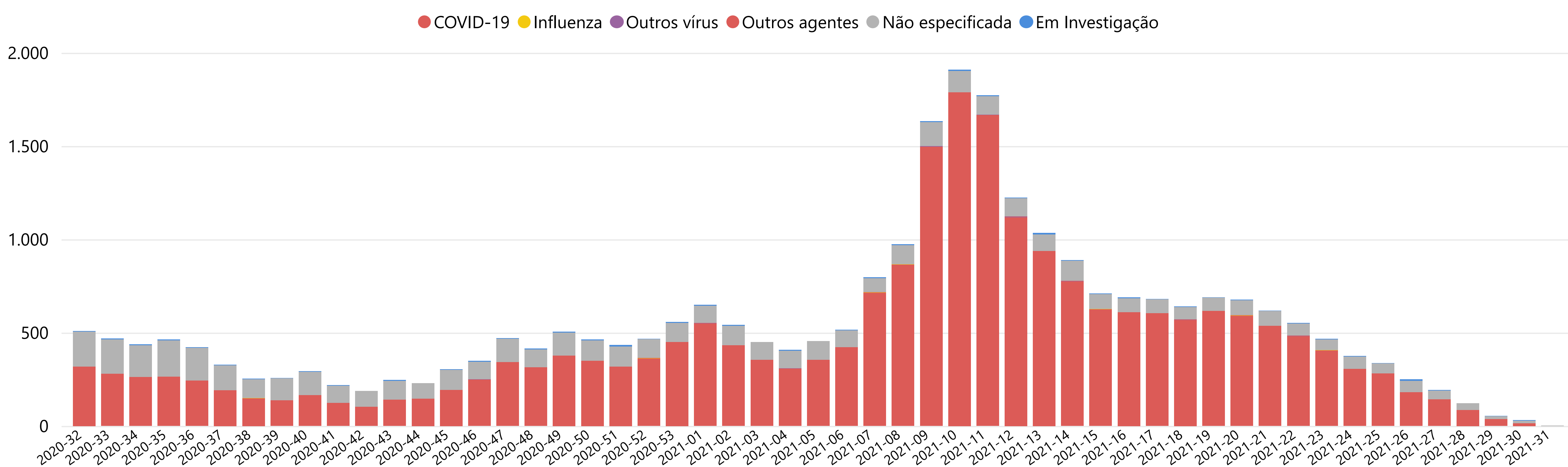
Óbitos por SRAG segundo semana epidemiológica de início de sintomas e classificação final. MSP, 08/08/2021
