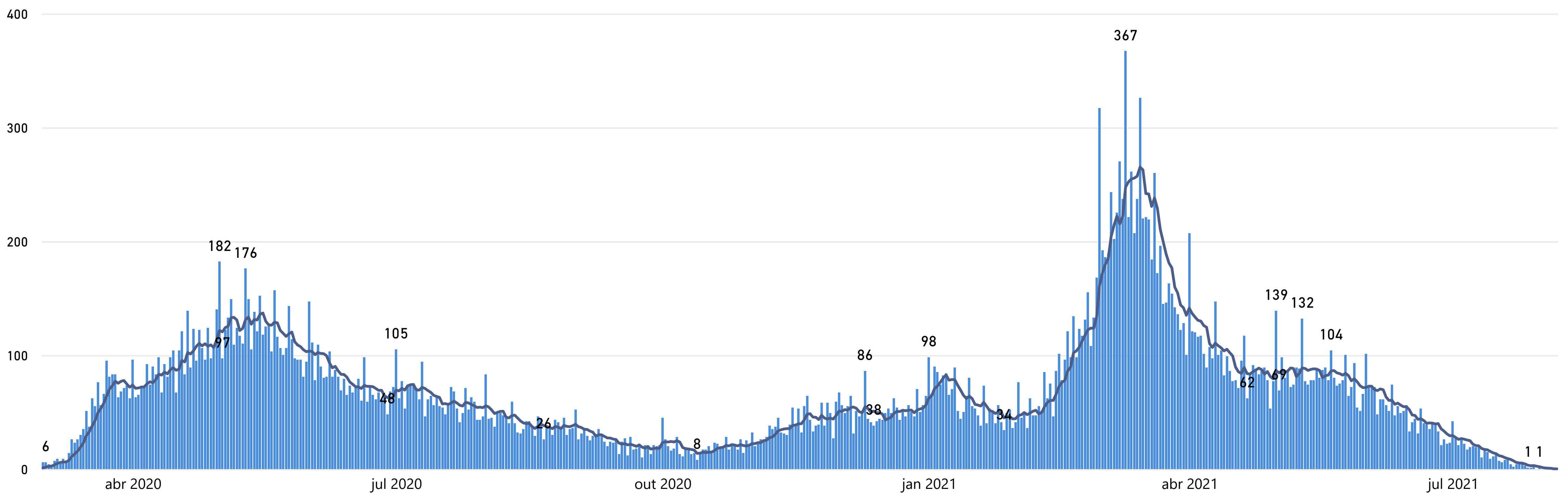
Óbitos confirmados para COVID-19 segundo data de início de sintomas. MSP, 08/08/2021
