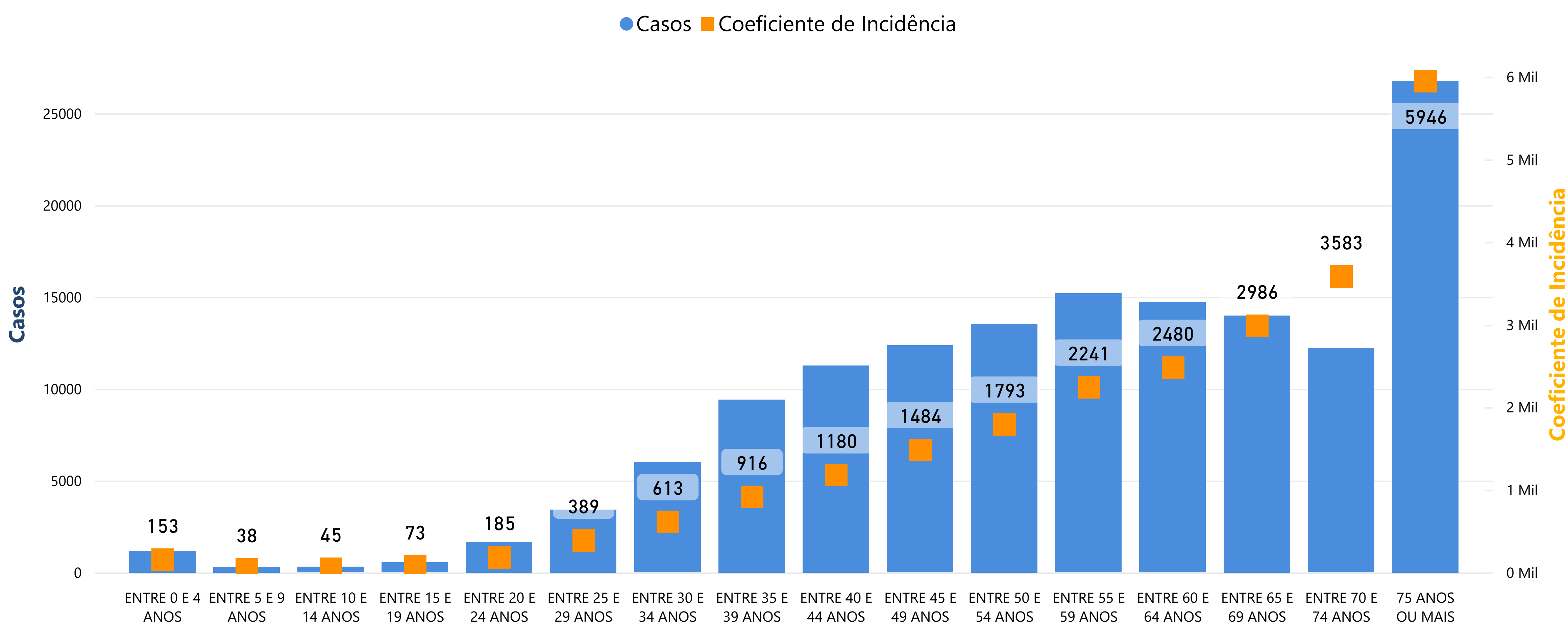
Casos de SRAG confirmados para COVID-19 e coeficiente de incidência por faixa etária. MSP, 08/08/2021
