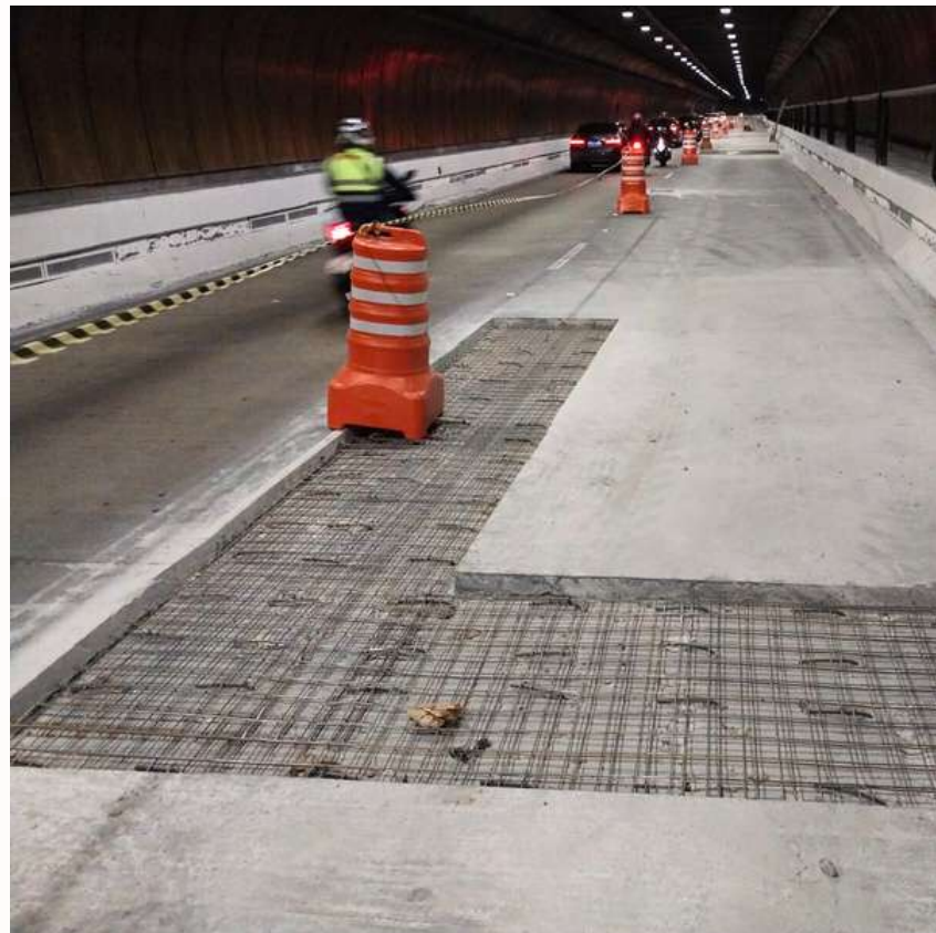
PAVIMENTO RÍGIDO - COMPLEXO VIÁRIO AYRTON SENNA
