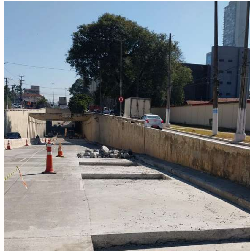
PAVIMENTO RÍGIDO - TÚNEL EUCLYDES DE JESUS ZERBINI
