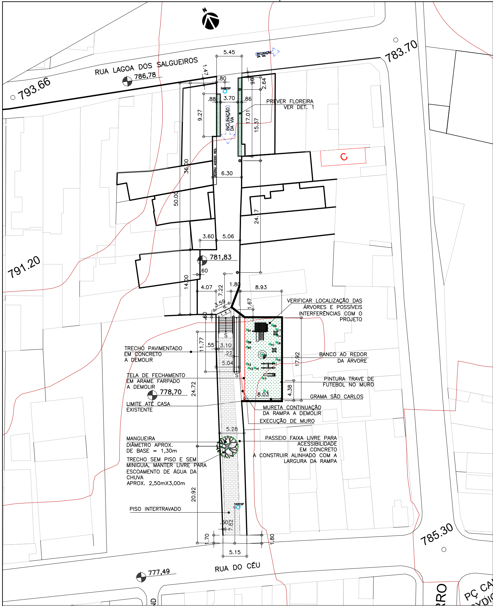
PLANTA GERAL ESCALA: 1:500
