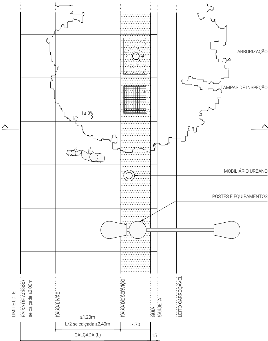
PLANTA
