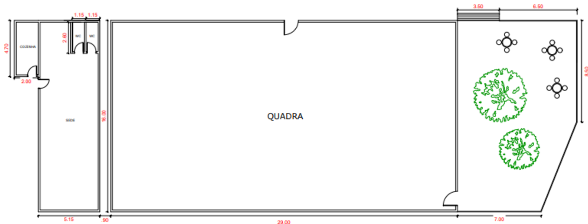
01 PLANTA BAIXA 1:50
