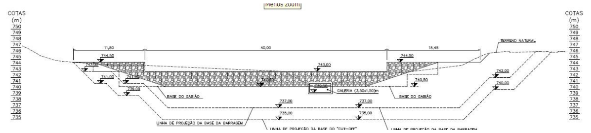
VISTA DE MONTANTE DA BARRAGEM R2 - s/escala
