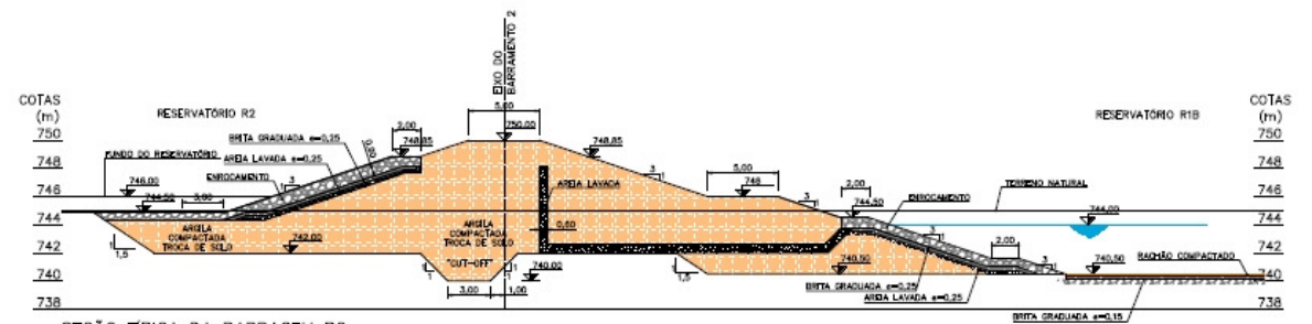
SEÇÃO TÍPICA DA BARRAGEM R2
