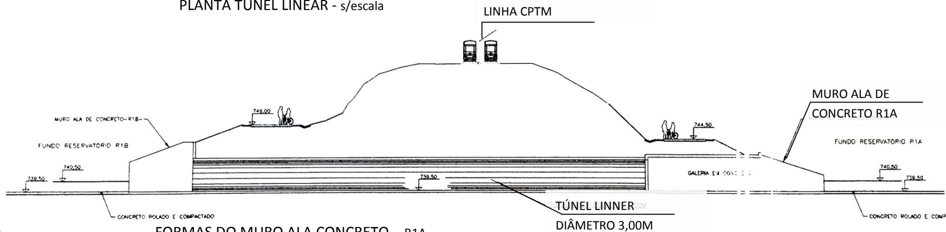
FORMAS DO MURO ALA CONCRETO – R1A
