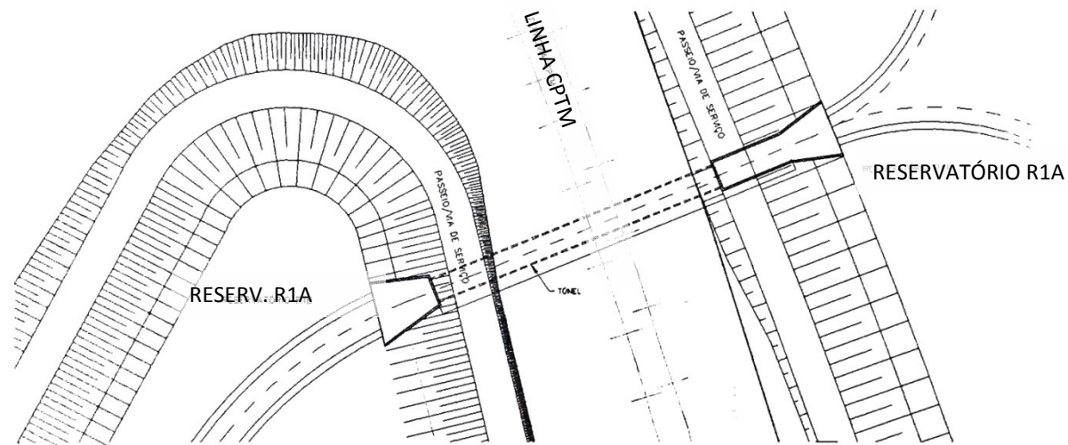
PLANTA TÚNEL LINEAR - s/escala
