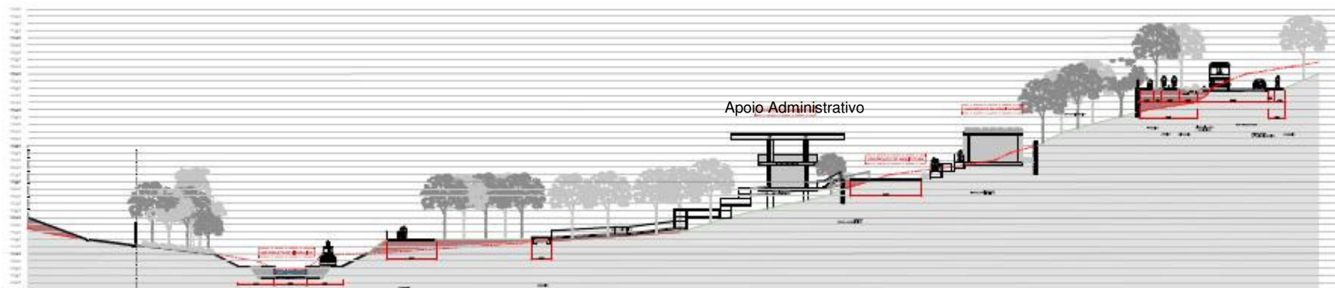
CORTE GERAL córrego
