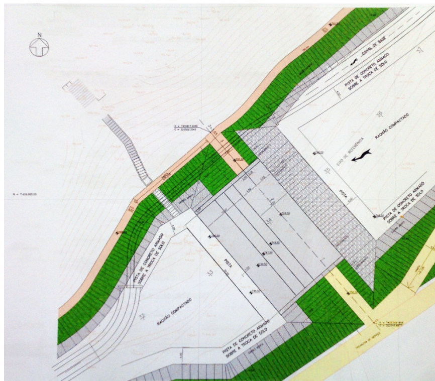
PLANTA BARRAGEM 1 - s/escala
