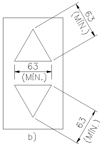
Figura 8 – Botões de Pavimento (Obs.: Medidas em milímetros)
