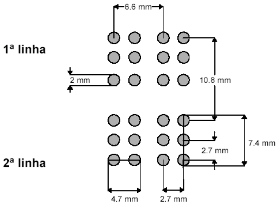
Figura 2 - Arranjo de 4 (quatro) células braille, distribuídas duas em cada linha
