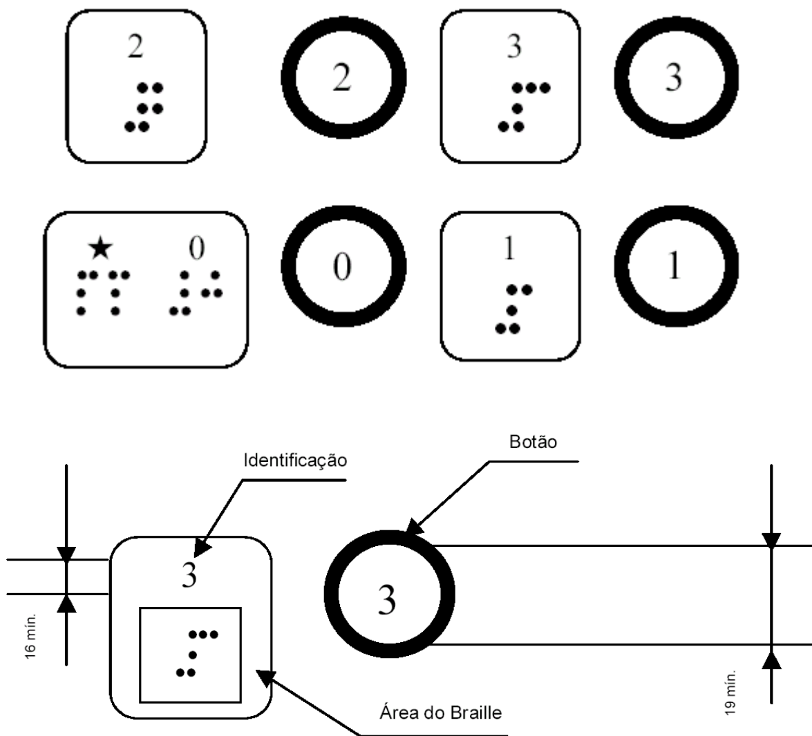
Figura 6 – Botão e sua identificação (Obs.: Medidas em milímetros)
