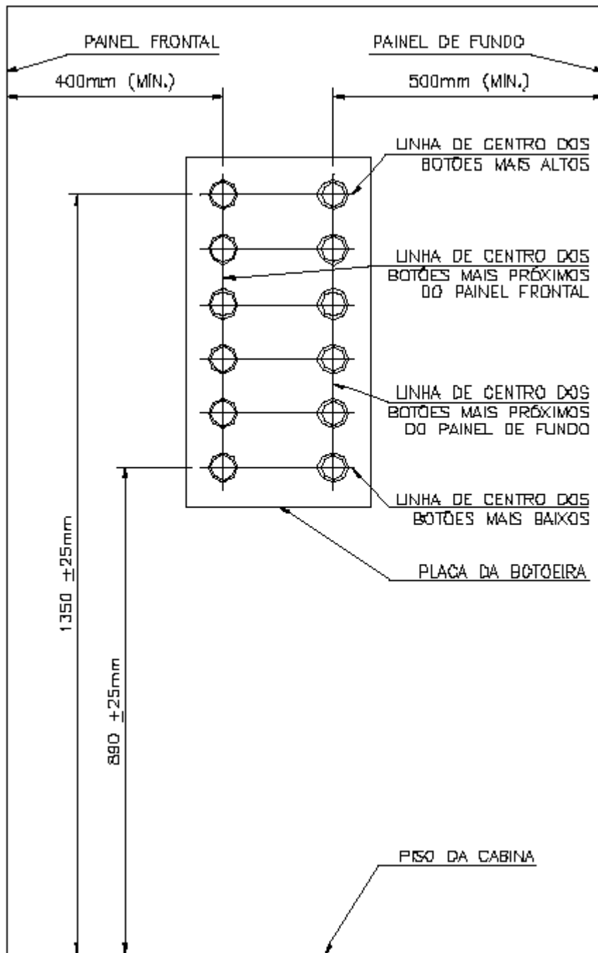
Figura 5 – Posicionamento de Botoeira da Cabina no Painel Lateral Direto (Obs.: Medidas em milímetros)
