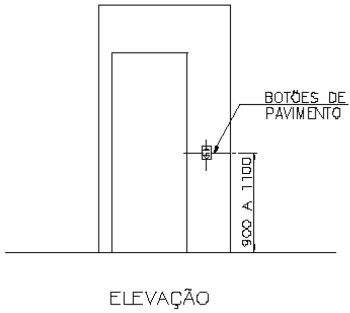
Figura 07 – Posicionamento dos Botões de Pavimento (Obs.: Medidas em milímetros)
