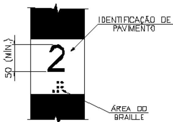
Figura 9 – Posicionamento das identificação de pavimentos (Obs.: Medidas em milímetros)
