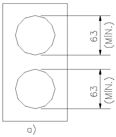
Figura 07 – Posicionamento dos Botões de Pavimento (Obs.: Medidas em milímetros)
