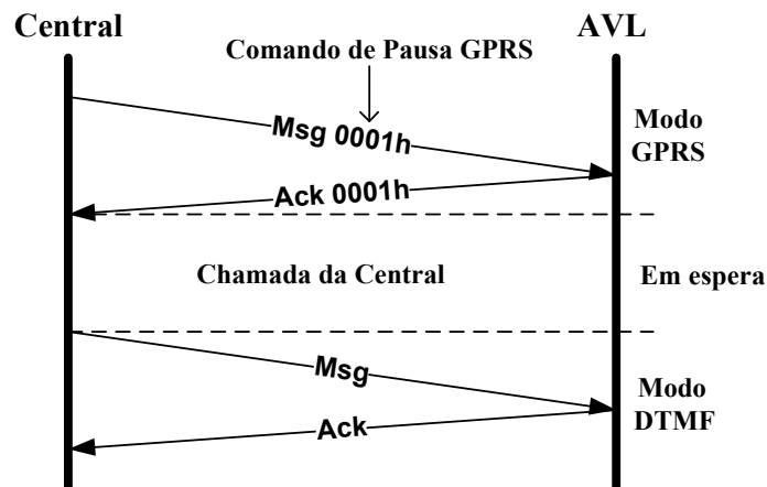
Figura 22 DTMF
