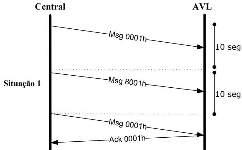
Figura 4 Seqüência sem Recepção
