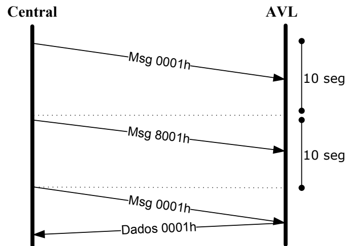
Figura 8 Seqüência Sem Recepção
