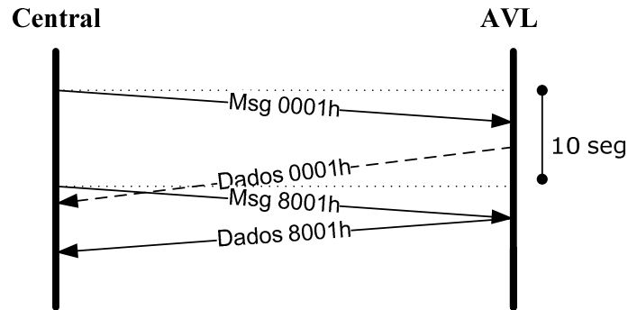
Figura 9 Seqüência com Atraso na Recepção
