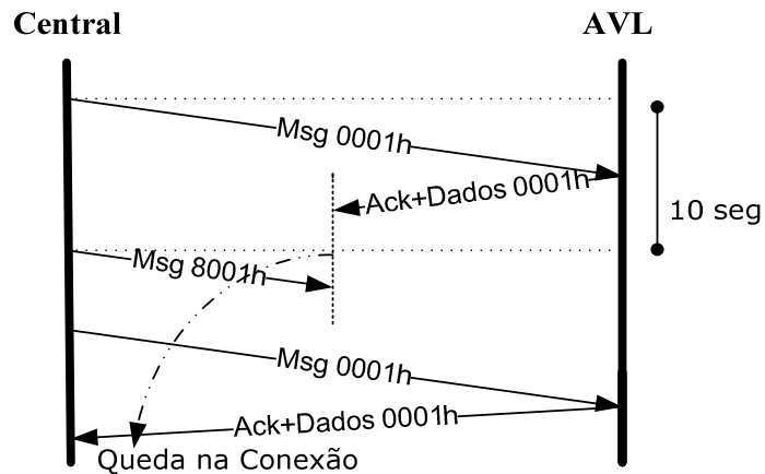
Figura 14 Sequência com Queda na Conexão
