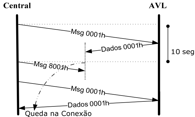
Figura 10 Sequência com Queda na Conexão
