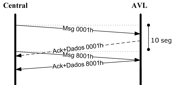
Figura 13 Seqüência com Atraso na Recepção
