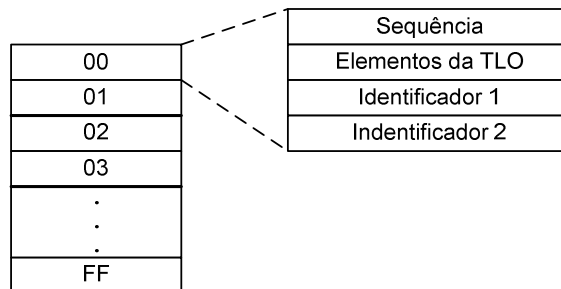
Figura 19 Estrutura de Carga de TLO
