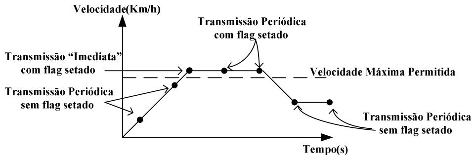
Figura 17 Excesso de Velocidade
