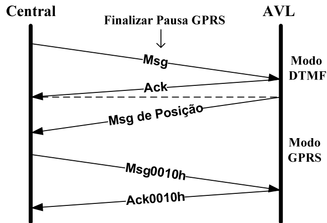
Figura 23 Finalização de Pausa GPRS
