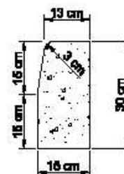
corte transversal
