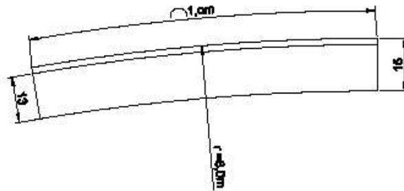
planta guia curva raio = 8,0m
