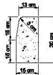
corte transversal
