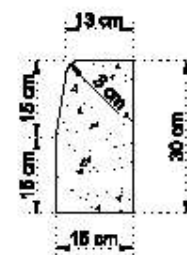
corte transversal
