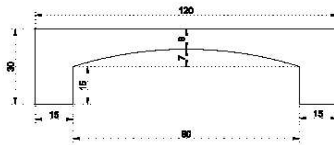
Elevação Guia Chapéu
