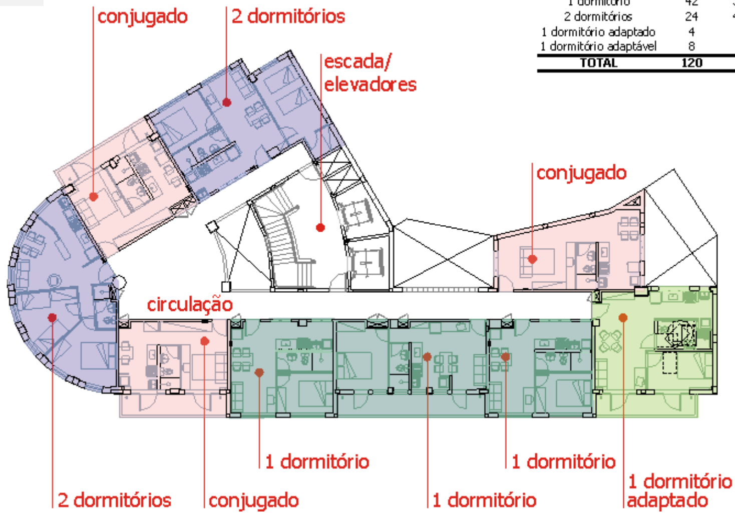
Pavimento Tipo
