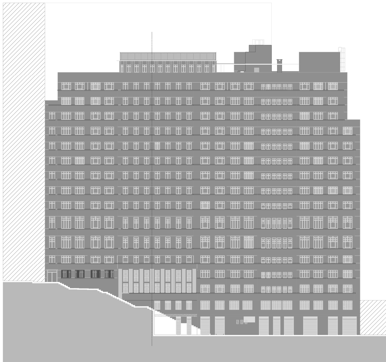
Fachada
