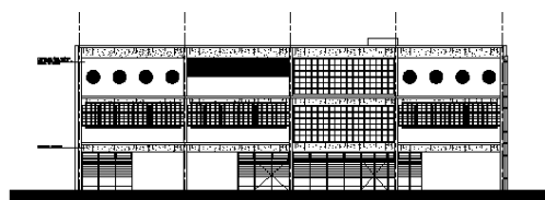
ELEVAÇÃO FRONTAL
