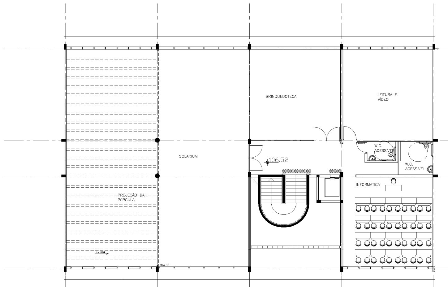
PLANTA DO SOLARIUM
