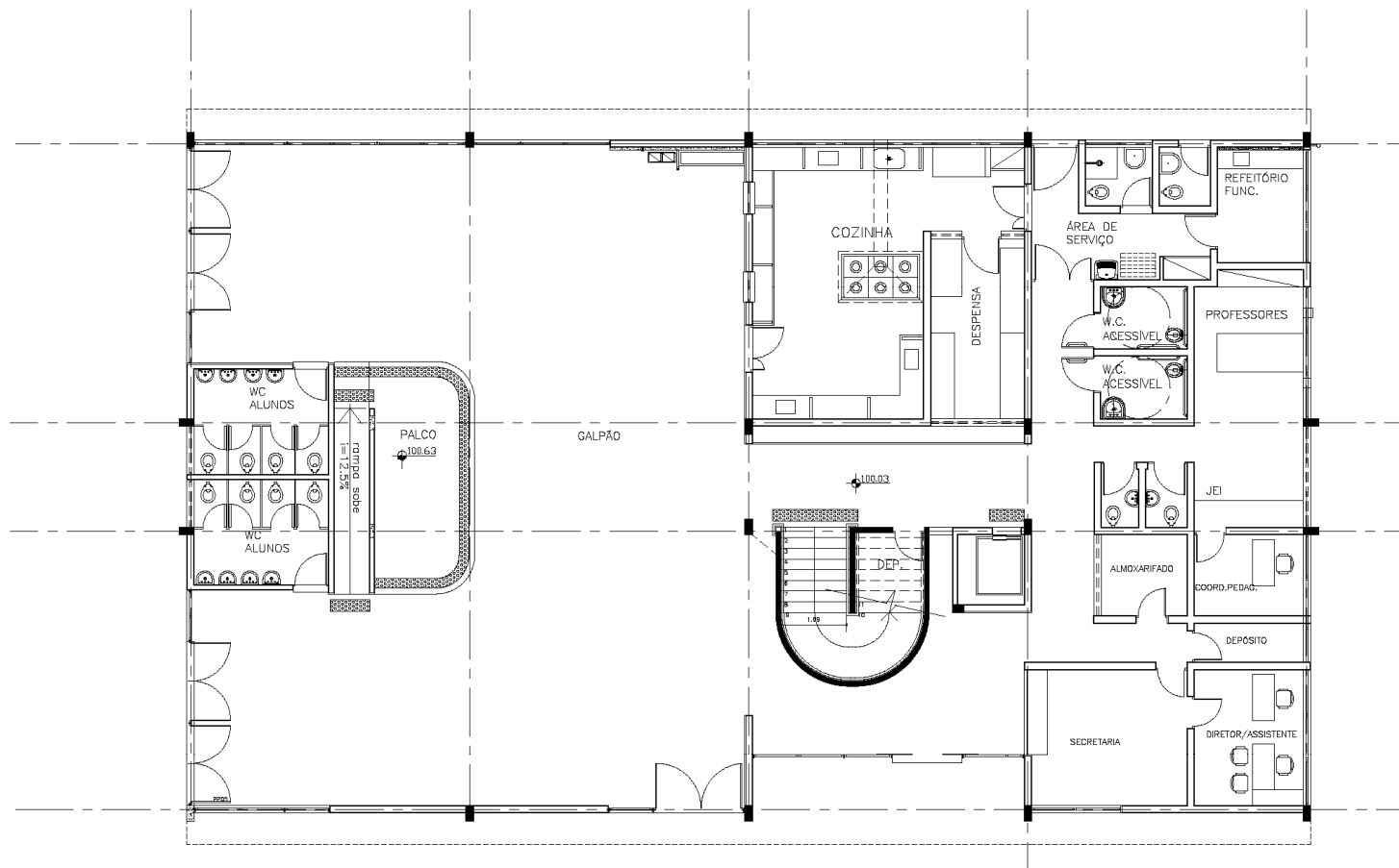
PLANTA PAV. TÉRREO
