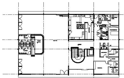
PLANTA PAV. TÉRREO
