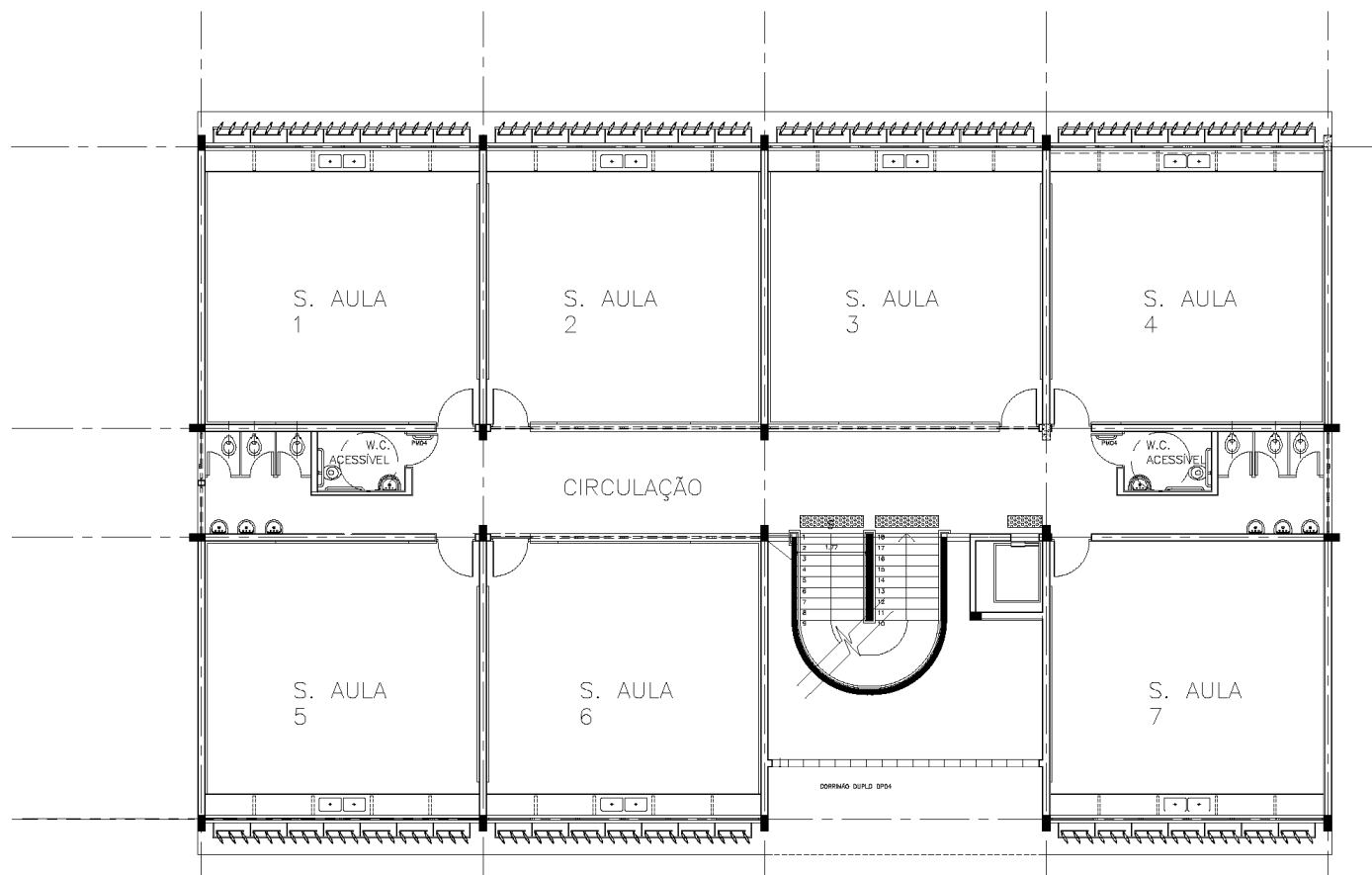
PLANTA PAV. SUPERIOR
