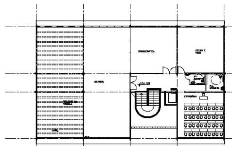
PLANTA DO SOLARIUM
