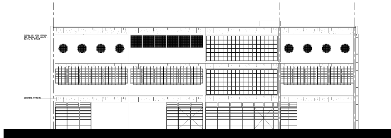
ELEVAÇÃO FRONTAL
