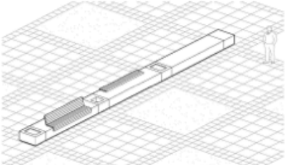
BANCO EM CONCRETO COM ASSENTO EM MADEIRA ISOMÉTRICA - ARTICULAÇÃO, EXEMPLO 1 ESCALA 1:10
