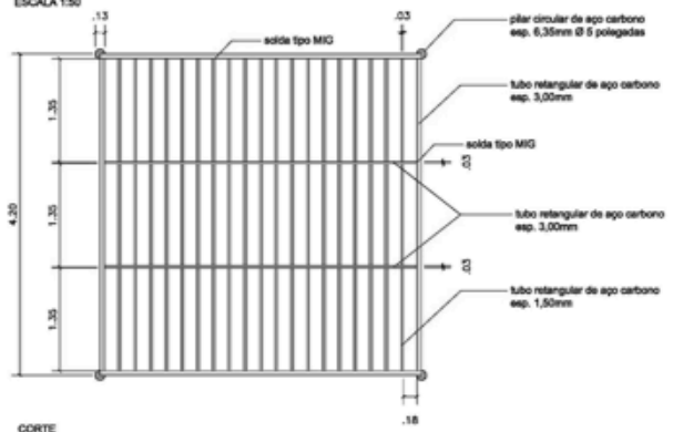
CORTE ESCALA 1:50
