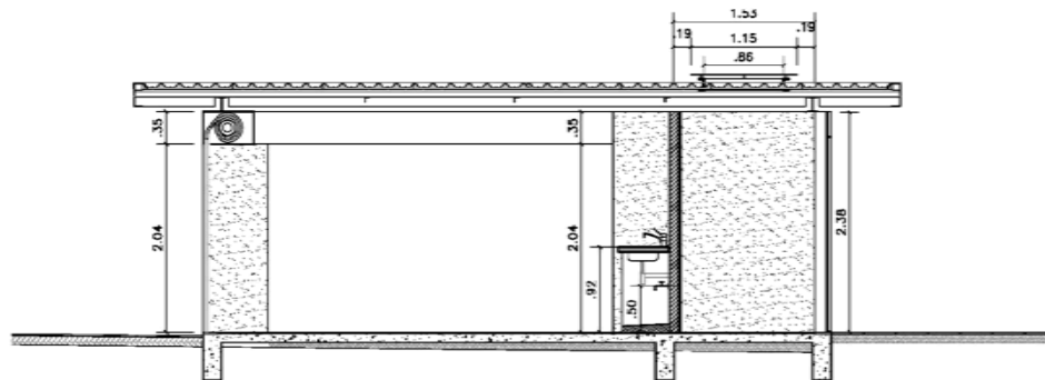
AMPLIAÇÃO - SANITÁRIO E QUIOSQUE CORTE AA ESCALA 1/50
