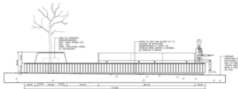
VISTA H ESCALA 1/20 MEDIDAS EM CM
