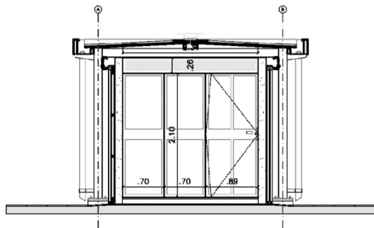
AMPLIAÇÃO - SANITÁRIO E QUIOSQUE CORTE BB ESCALA 1/50
