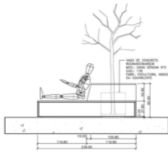
VISTA G ESCALA 1/20 MEDIDAS EM CM
