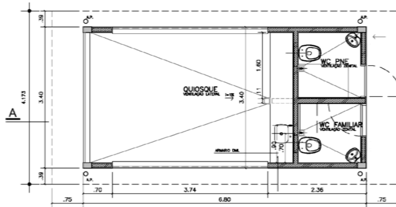
AMPLIAÇÃO - SANITÁRIO E QUIOSQUE PLANTA ESCALA 1/50
