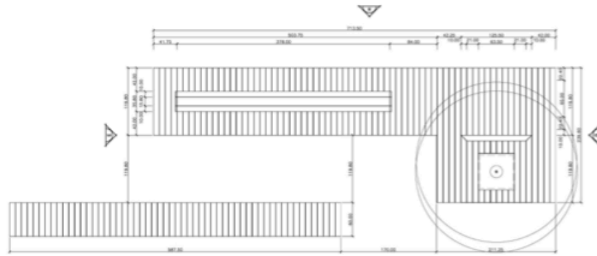
INPLANTAÇÃO DO BANCO ILHA ESCALA 1/20 MEDIDAS EM CM
