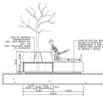
VISTA E ESCALA 1/20 MEDIDAS EM CM
