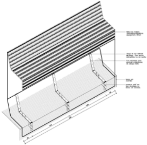
ESQUEMA DE MONTAGEM DO BANCO - ISOMÉTRICA ESCALA 1:10 O BANCO É FORMADO POR MÓDULOS DE 0,70m DE ALTEZURA TOTAL (0,40m DE CONCRETO + 0,30m DE MADEIRA). O MÓDULO DE 0,70m APRESENTA ANOSOS PARA O PISO DE PLÁSTICO, INCLINADO 2°.
